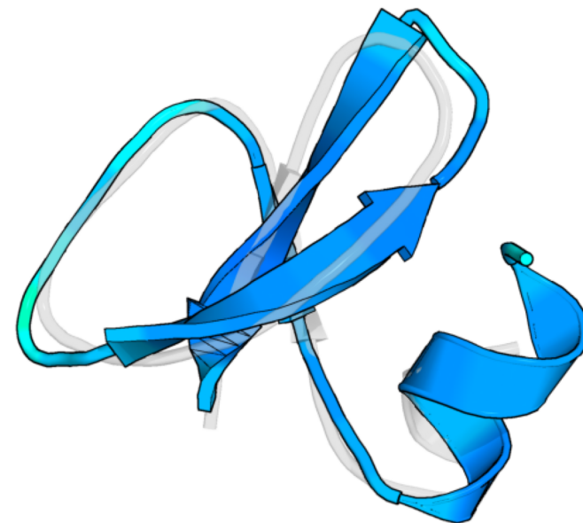
Defensin_beta
