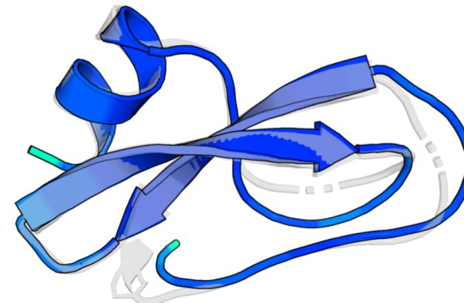
Kunitz
