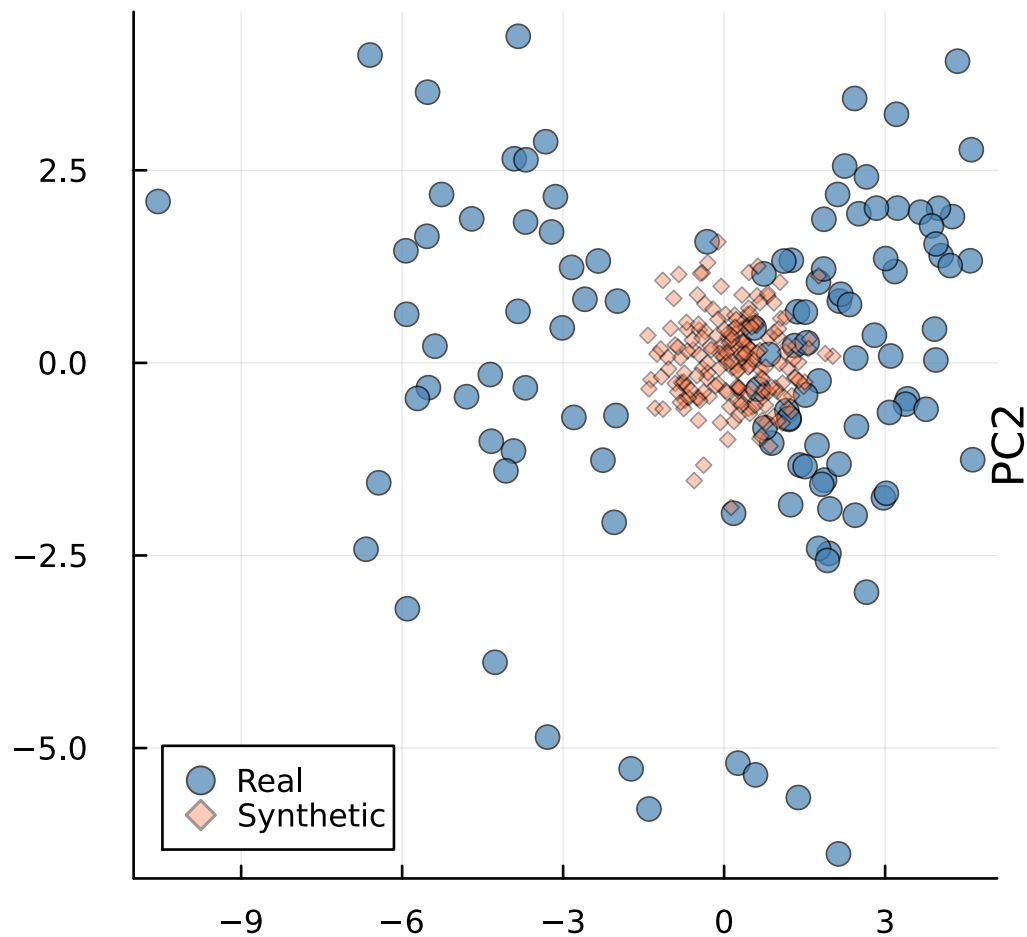
A: Unit-Norm
