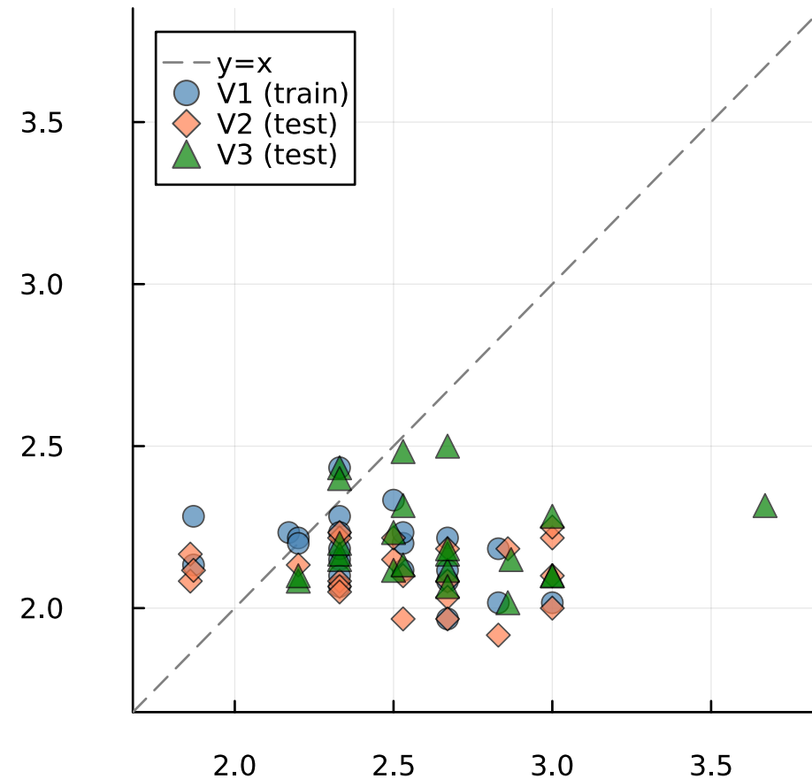
Lagtime (min)
