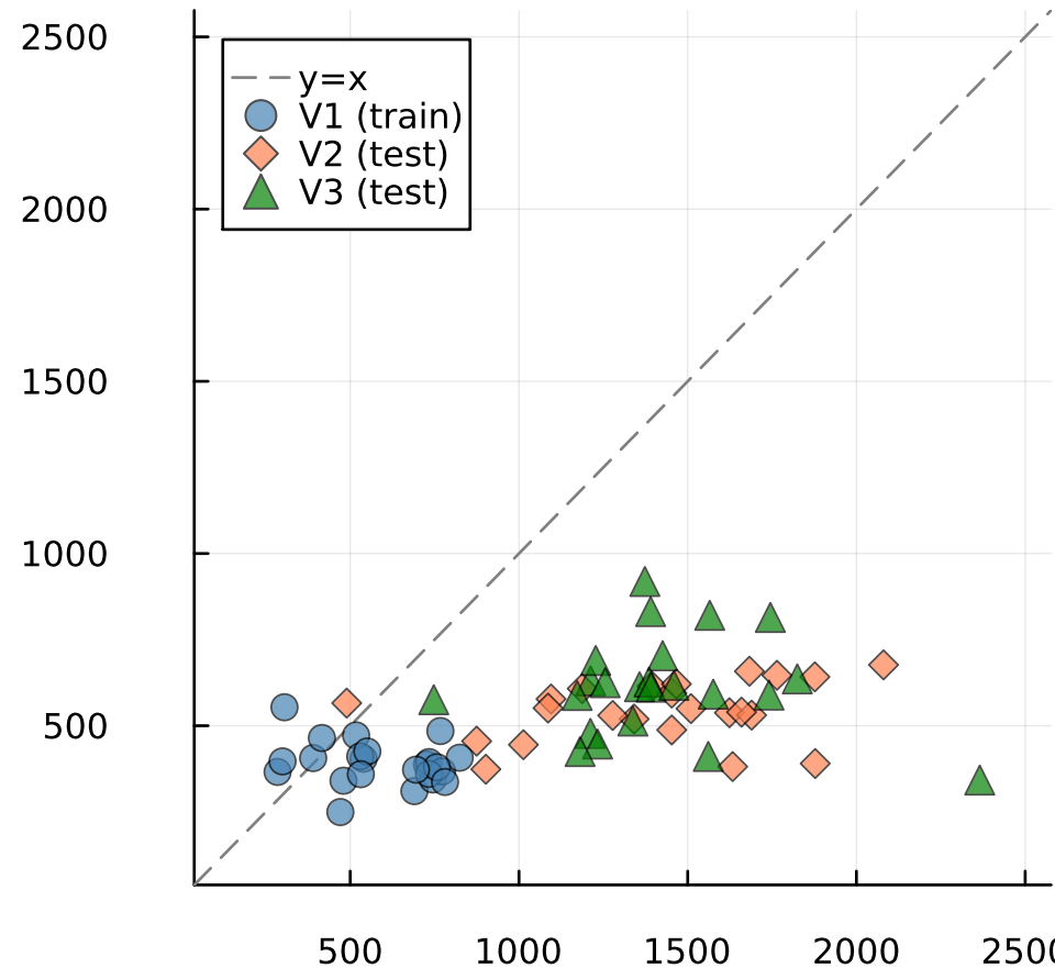
ETP (nM·min)
