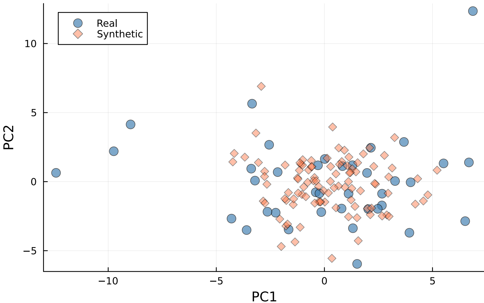
Longitudinal PCA: Real vs Synthetic ( K=38 , d=27 )
