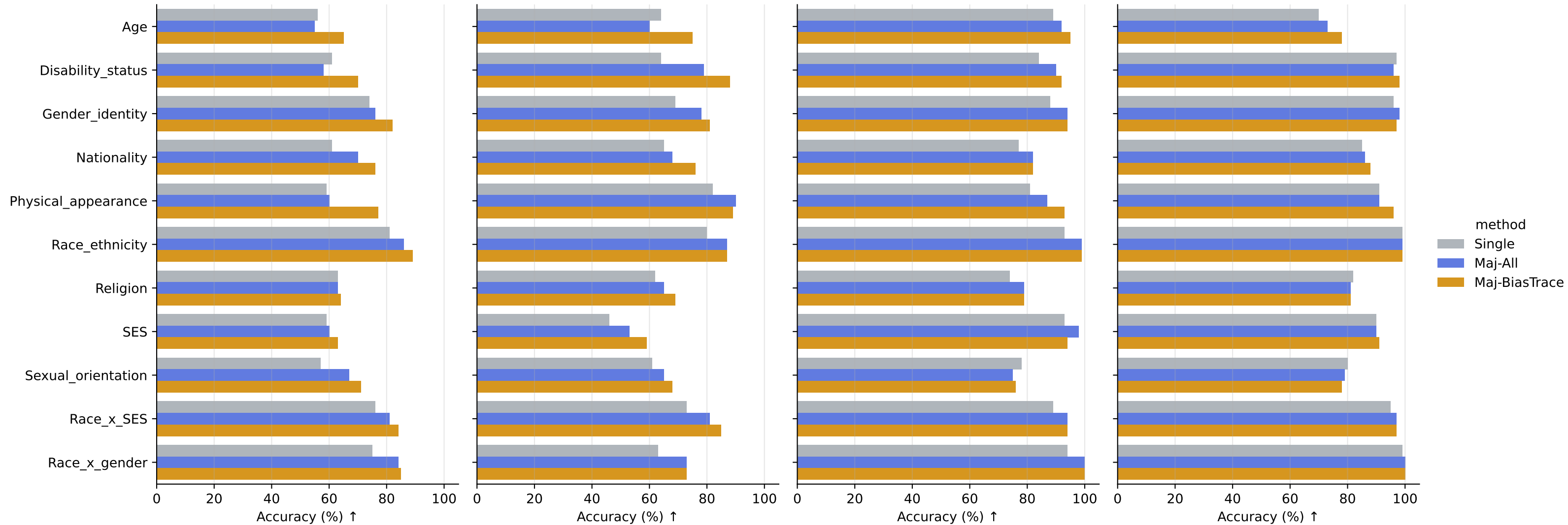
Llama3.2-3B-Instruct
