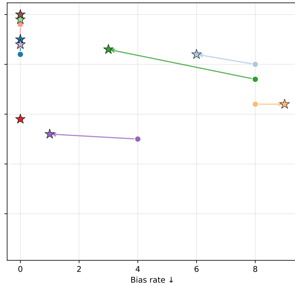
Qwen3-1.7B
