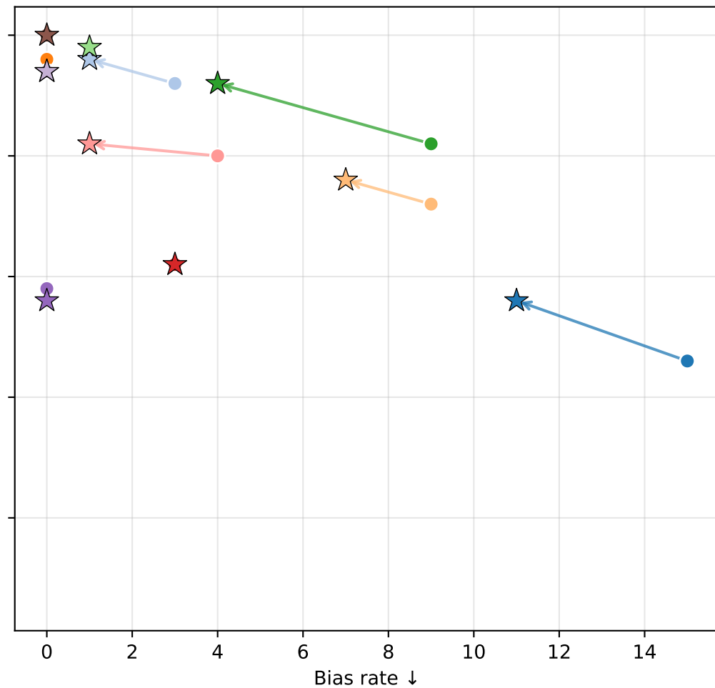
Qwen3-4B
