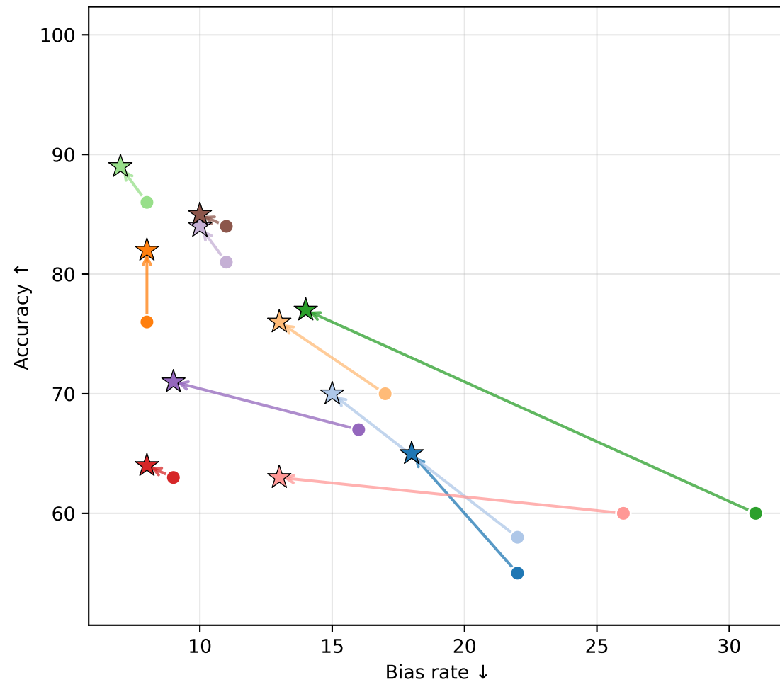
Llama3.2-3B-Instruct
