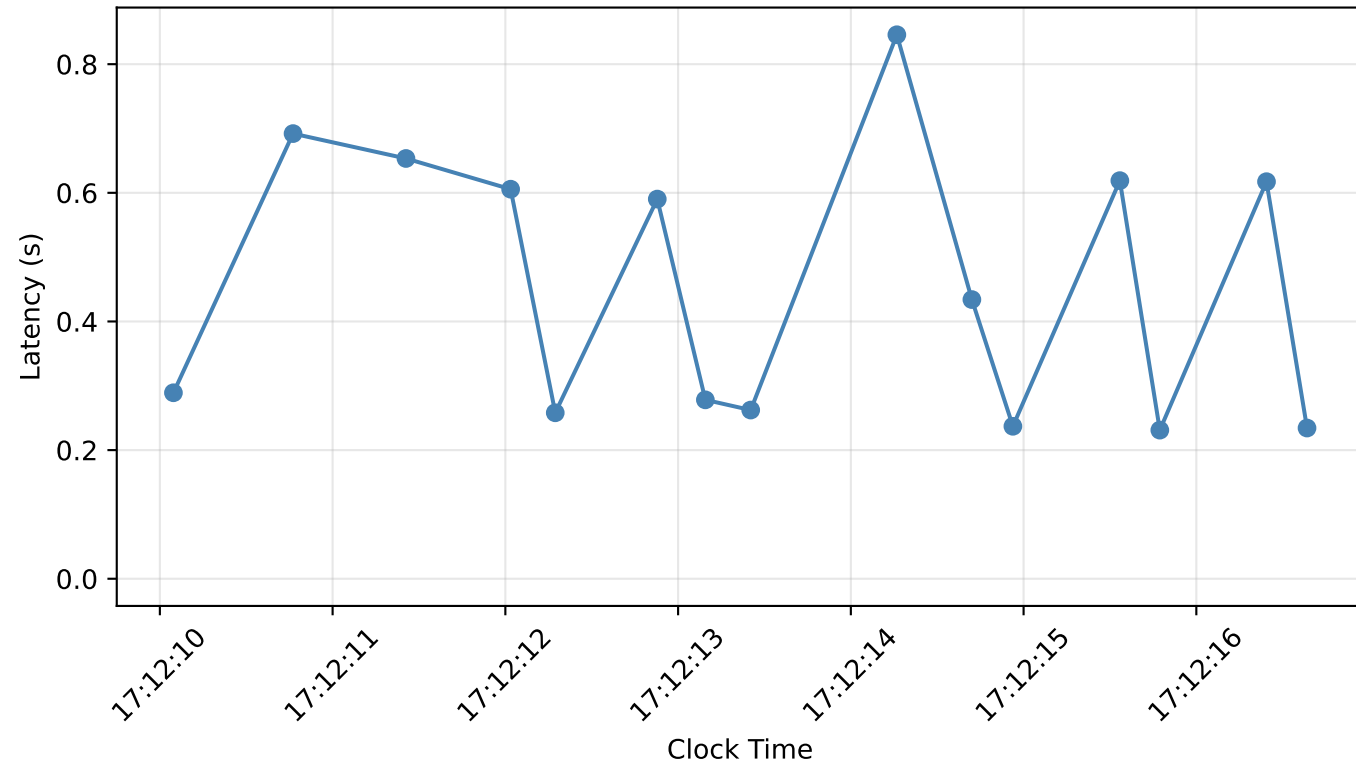
CEDA
