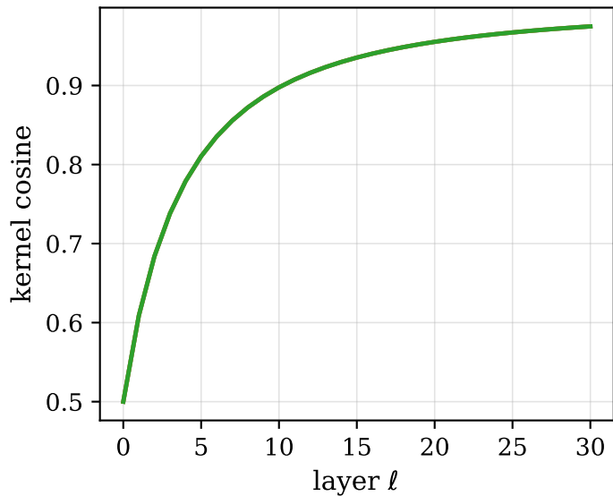
init c = 0.5
