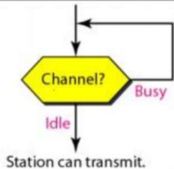
a. 1-persistent
