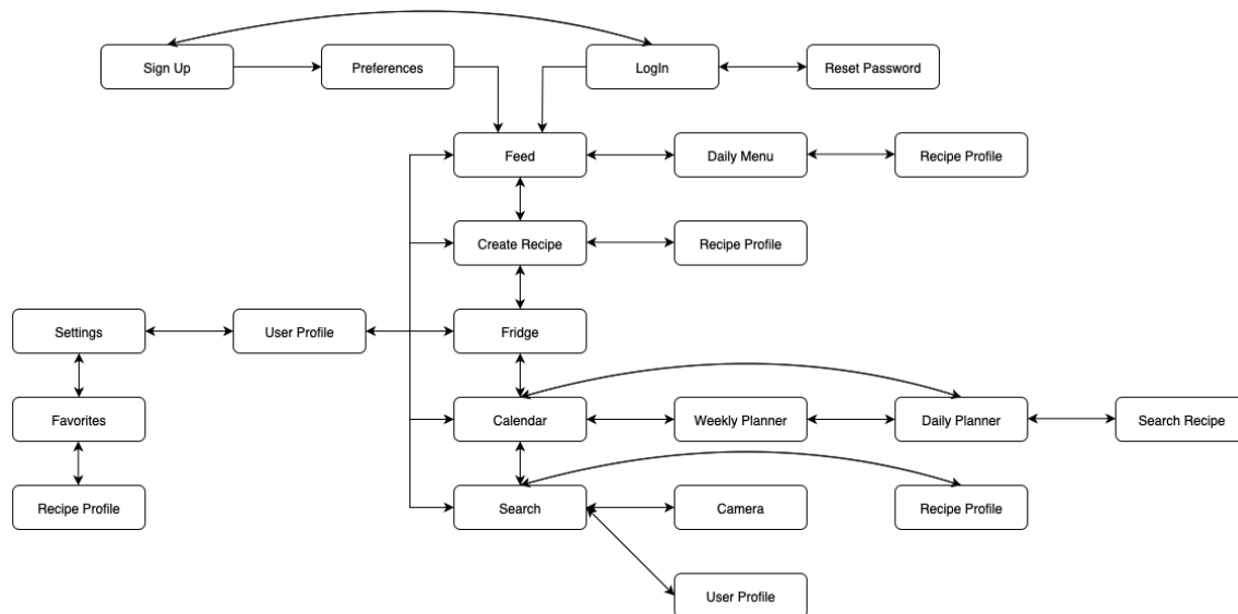
Figura 5.1: Grafo de navegação da aplicação
