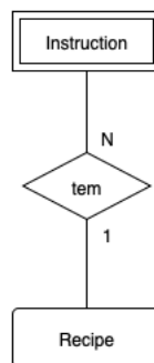
Figura 3.5: Diagrama Entidade-Associação de Instruction
