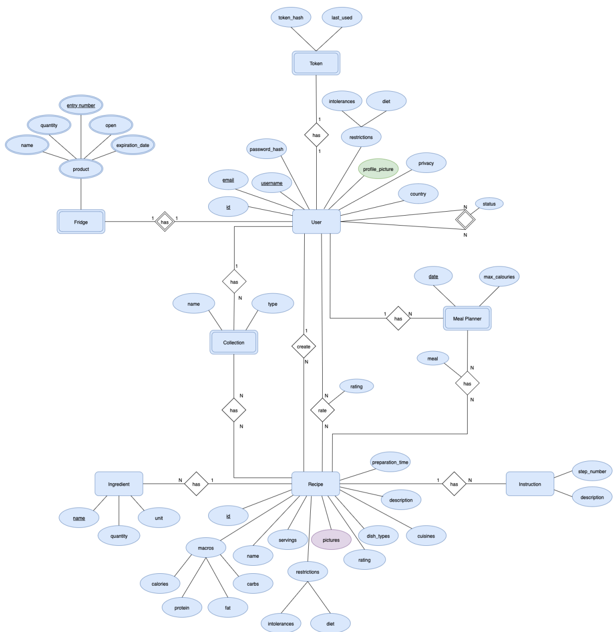
Figura A.1: Modelo Entidade-Associação
