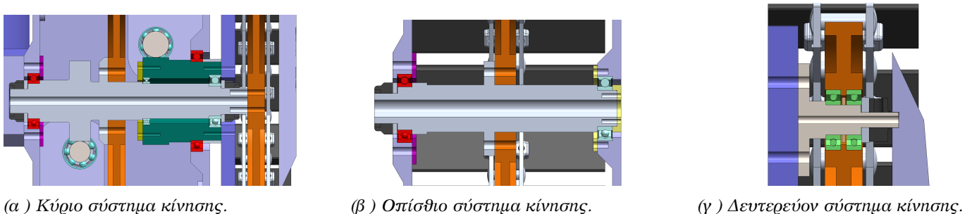
Σχήμα 2.46: Τομές συναρμολογημένων διατάξεων συστημάτων κίνησης κατά τη δεύτερη επανάληψη του ισοζυγίου μάζας v2.
