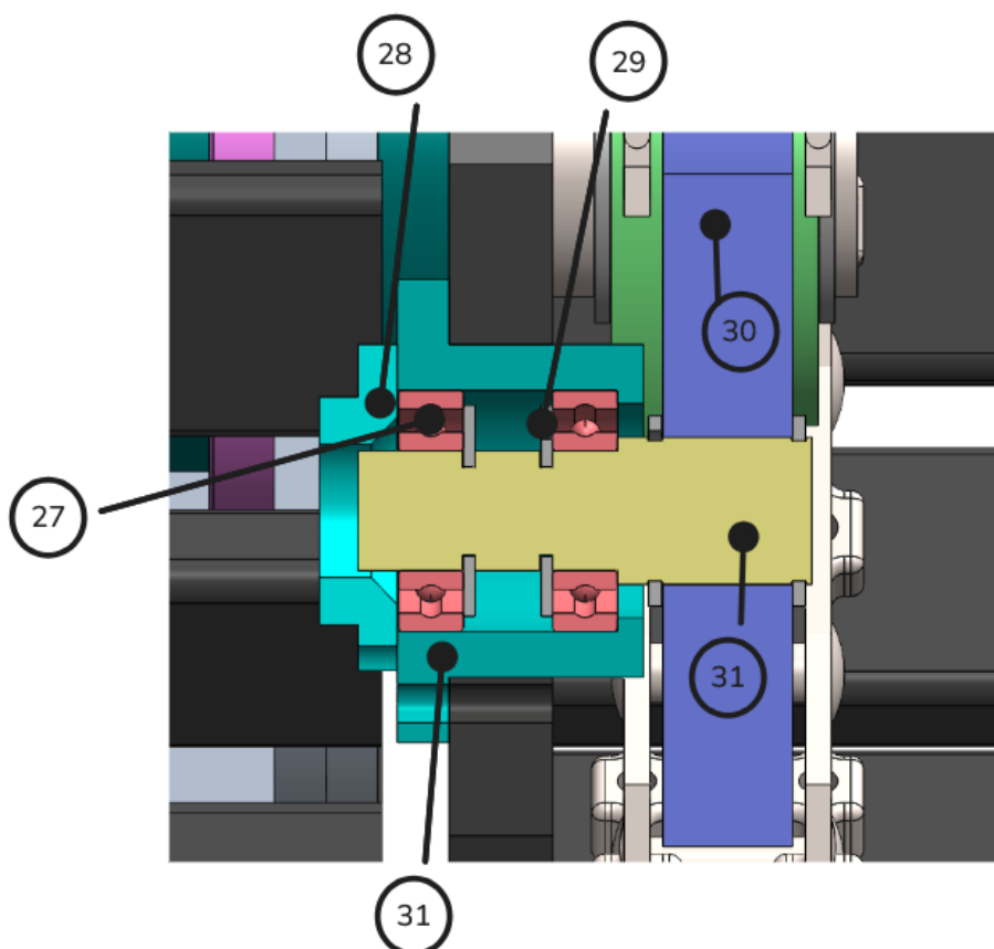
Σχήμα 2.25: Τομή συναρμολογημένης διάταξης δευτερέων συστήματος κίνησης v1.
