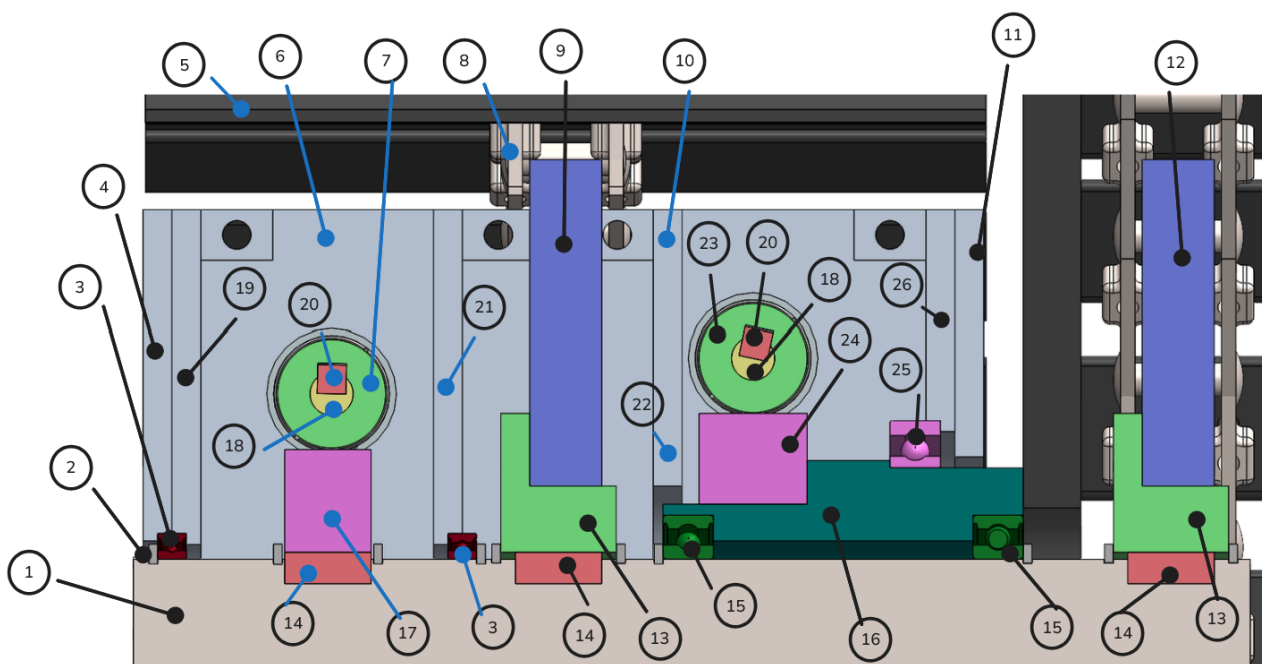
Σχήμα 2.24: Τομή συναρμολογημένης διάταξης κύριου συστήματος κίνησης v1.
