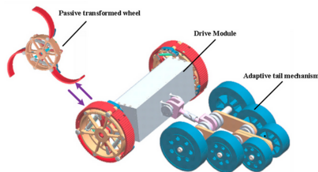
(β) Σύστημα μεταβλητής γεωμετρίας τροχού [16].
