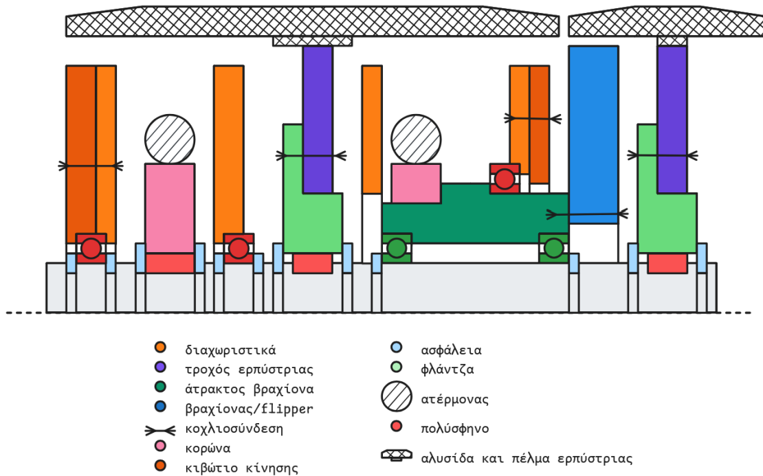
Σχήμα 2.15: Αρχικό σκαρίφημα κιβωτίου κίνησης.
