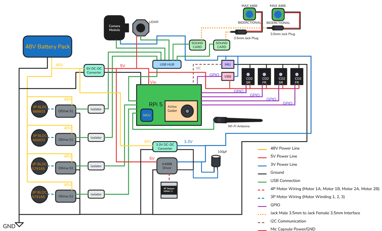
Σχήμα 2.57: Κύκλωμα ηλεκτρονικών.
