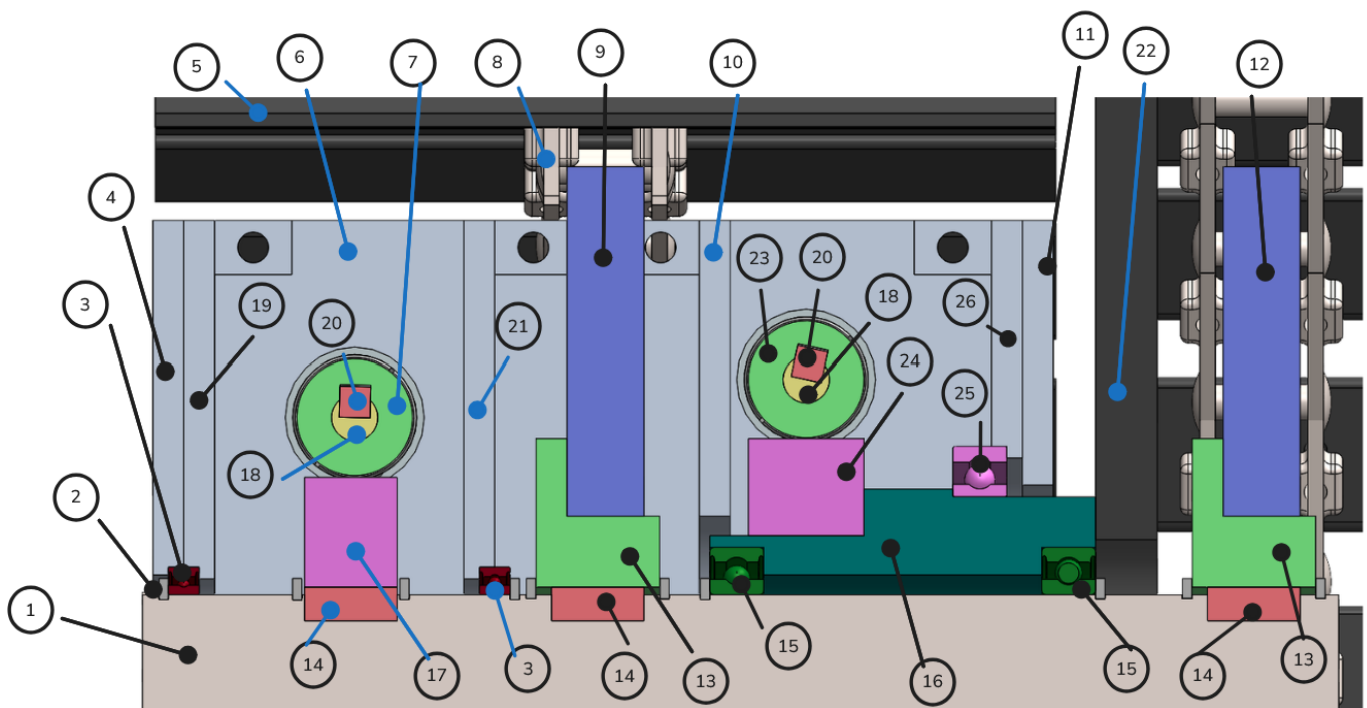
Σχήμα 2.26: Τομή συναρμολογημένης διάταξης κύριου συστήματος κίνησης v1.
