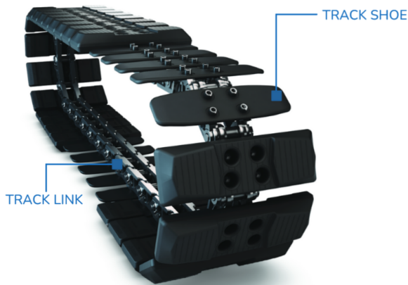
(α ) Ερπύστρια με αρθρωτούς συνδέσμους.
