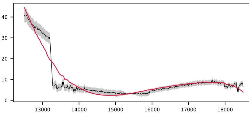
-621235758478664148, 2.1' S/N 54, LSF 22 Å, GALAXY, z = 0.200 , \Delta\chi^2=3 , \chi^2_r=1.9
