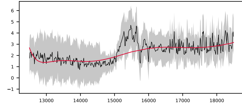
-620881463478533288, 2.7' S/N 16, LSF 13 Å, GALAXY, v = +0 \text{ km/s} , \Delta\chi^2=0 , \chi^2_r=1.6
