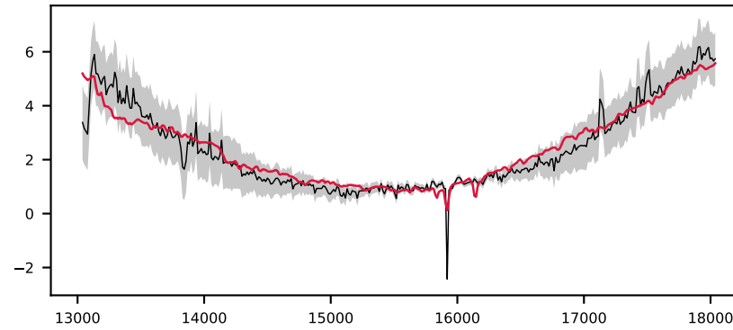
-622926396479361410, 8.1' S/N 15, LSF 33 Å, GALAXY, z = 0.041 , \Delta\chi^2=17 , \chi^2_{\text{r}}=0.9
