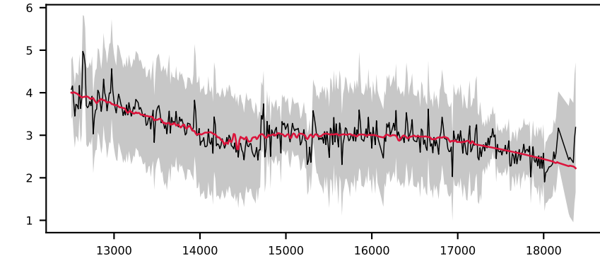
-620879278479317711, 2.1' S/N 25, LSF 18 Å, GALAXY, z = 0.189 , \Delta\chi^2=20 , \chi^2_r=5.4
