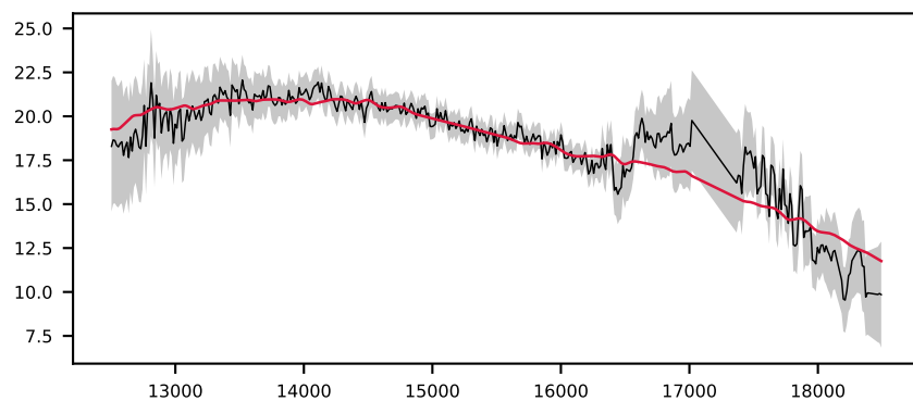
-621541444478953065, 2.2' S/N 56, LSF 39 Å, GALAXY, z = 0.096 , \Delta\chi^2=4 , \chi^2_r=0.4
