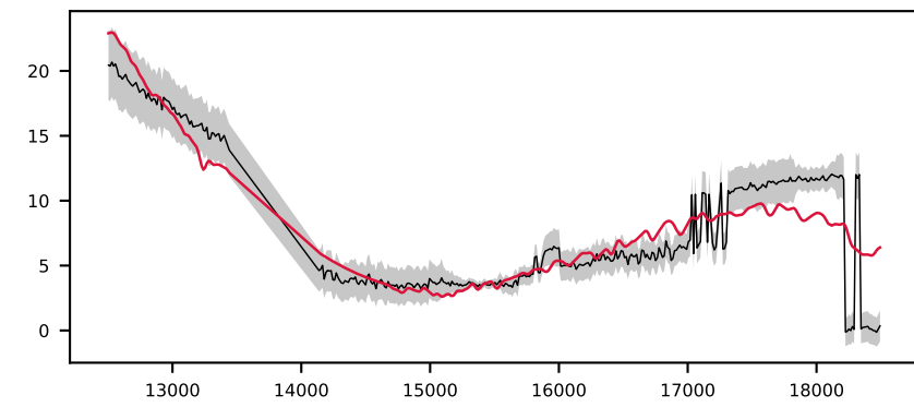
-620638526479232535, 2.2' S/N 47, LSF 18 Å, GALAXY, z = 0.244 , \Delta\chi^2=10 , \chi^2_r=0.3
