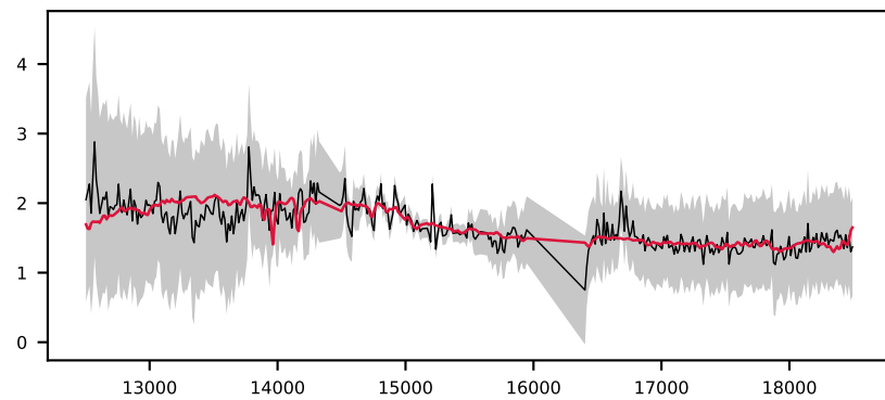
-622915563478725797, 7.8' S/N 14, LSF 19 Å, GALAXY, z = 0.999 , \Delta\chi^2=50 , \chi^2_{\text{r}}=0.4
