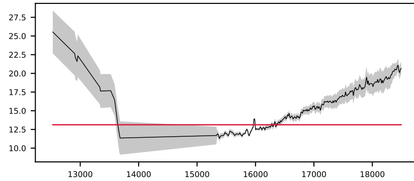
-621306707478711783, 2.0' S/N 85, LSF 14 Å, GALAXY, z = 0.304 , \Delta\chi^2=46 , \chi^2_r=1.3
