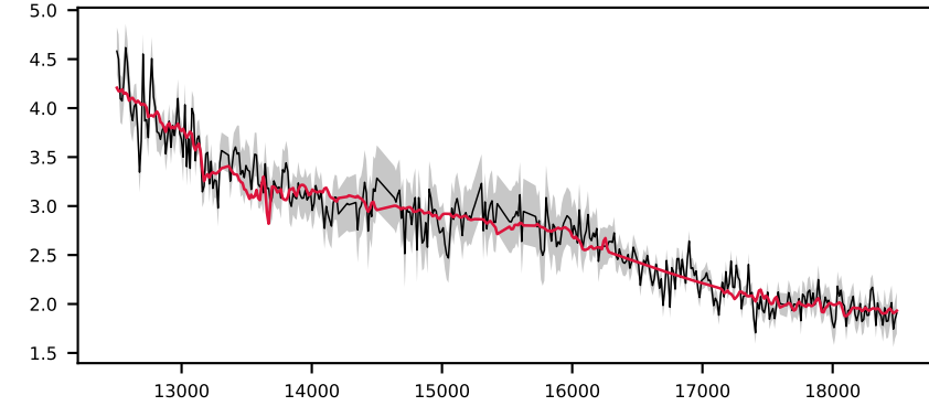
-621283886479253499, 2.0' S/N 23, LSF 16 Å, GALAXY, z = 0.056 , \Delta\chi^2=12 , \chi^2_r=0.7
