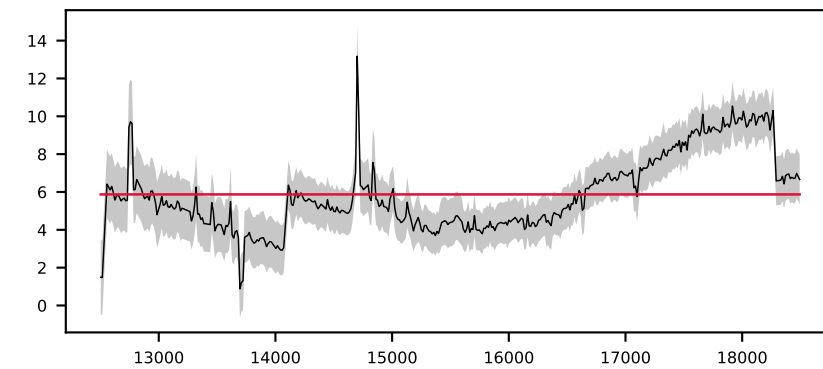
-621065576479280108, 1.9' S/N 40, LSF 27 Å, GALAXY, z = 0.054 , \Delta\chi^2=57 , \chi^2_r=4.1
