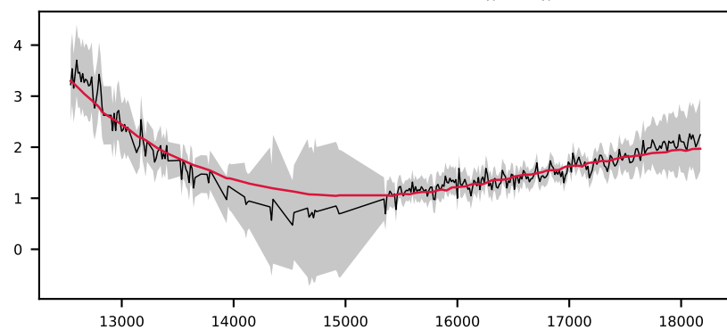
-619367398479083997, 6.6' S/N 13, LSF 16 Å, GALAXY, z = 0.047 , \Delta\chi^2=5 , \chi^2_r=0.5
