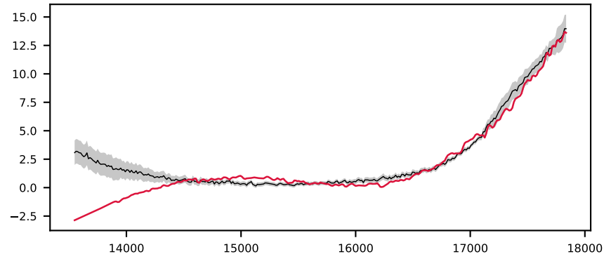
-622167476479795735, 6.8' S/N 13, LSF 12 Å, GALAXY, z = 0.282 , \Delta\chi^2=13 , \chi^2_r=1.0
