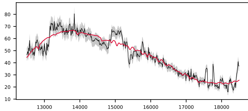
-620927162479187773, 1.3' S/N 108, LSF 13 Å, GALAXY, z = 0.203 , \Delta\chi^2=58 , \chi^2_r=9.6
