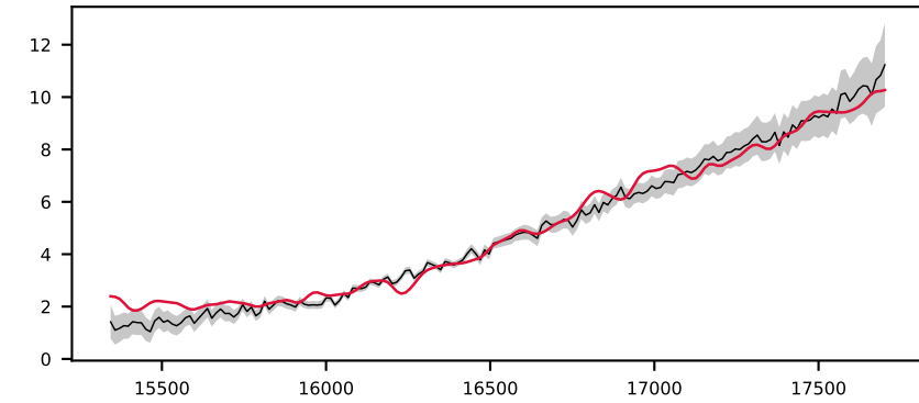
-620918583478289770, 4.1' S/N 32, LSF 12 Å, GALAXY, z = 0.208 , \Delta\chi^2=8 , \chi^2_r=0.4
