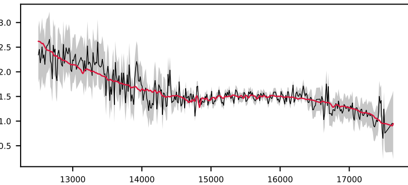
-622112542479339050, 5.0' S/N 15, LSF 13 Å, GALAXY, z = 0.308 , \Delta\chi^2=2 , \chi^2_{\text{r}}=0.6
