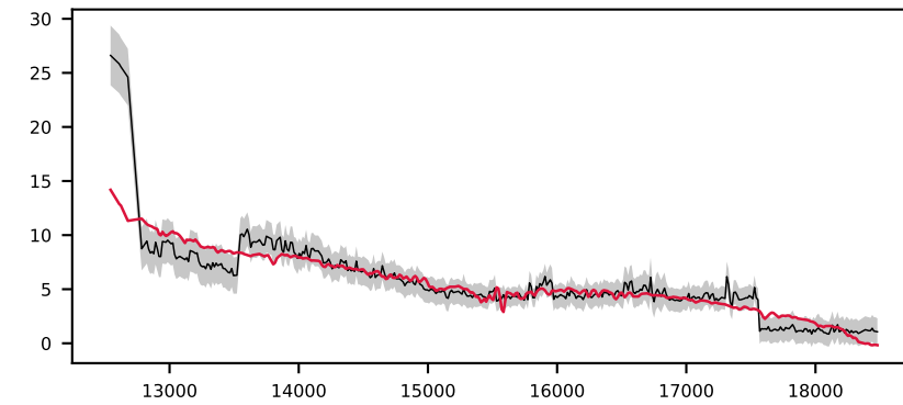
-621142691479279694, 1.9' S/N 39, LSF 21 Å, GALAXY, z = 0.048 , \Delta\chi^2=23 , \chi^2_r=2.2
