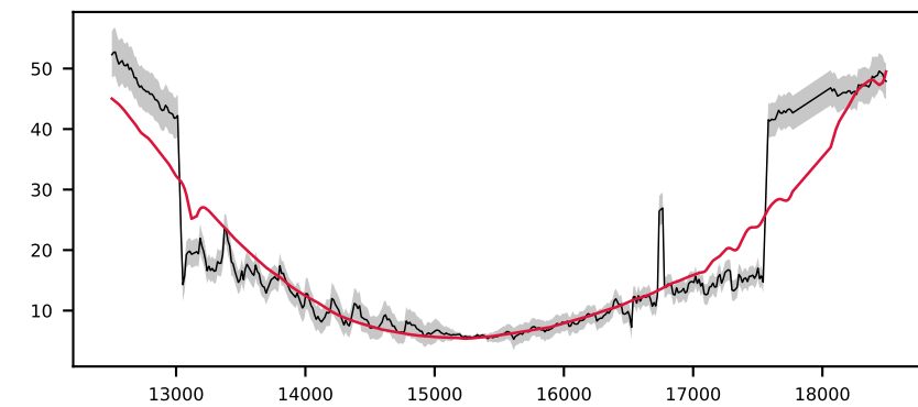
-620743995478758227, 1.6' S/N 74, LSF 13 Å, GALAXY, z = 0.093 , \Delta\chi^2=8 , \chi^2_r=3.2
