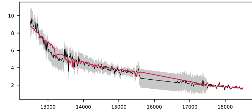
-622921362478652715, 7.9' S/N 31, LSF 11 Å, GALAXY, z = 0.059 , \Delta\chi^2=2 , \chi^2_r=0.2
