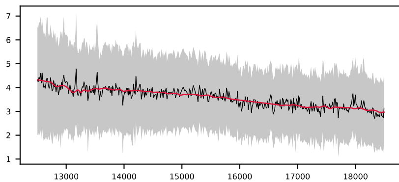
-618622144479050663, 9.6' S/N 22, LSF 26 Å, GALAXY, z = 0.168 , \Delta\chi^2=0 , \chi^2_{\text{r}}=0.0
