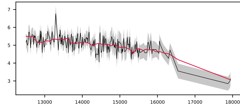
-619989119478871243, 4.1' S/N 23, LSF 14 Å, GALAXY, z = 0.248 , \Delta\chi^2=2 , \chi^2_r=0.9
