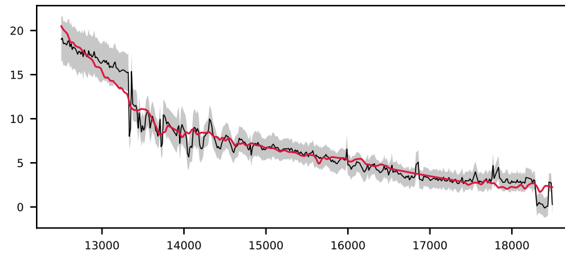
-621427871478728495, 2.2' S/N 44, LSF 26 Å, GALAXY, z = 0.331 , \Delta\chi^2=82 , \chi^2_r=0.5
