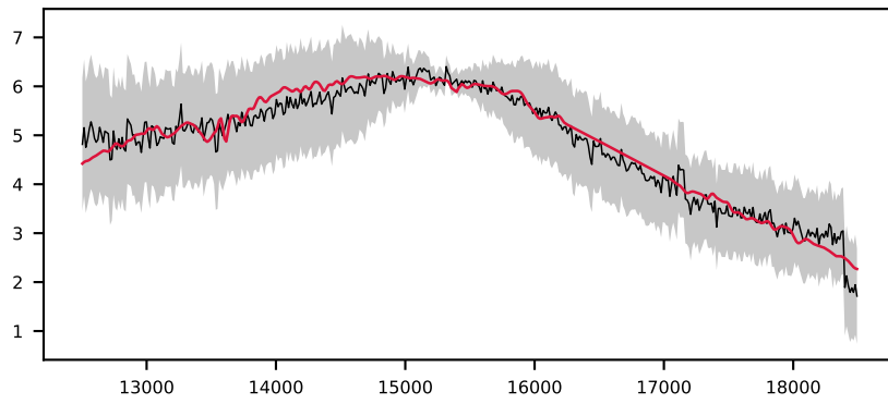
-621998362478530332, 4.8' S/N 45, LSF 21 Å, GALAXY, z = 0.205 , \Delta\chi^2=1 , \chi^2_r=0.8
