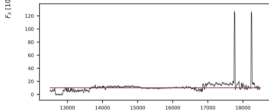
-621447045480055097, 6.7' S/N 74, LSF 12 Å, GALAXY, z = 0.343 , \Delta\chi^2=5 , \chi^2_r=0.8
