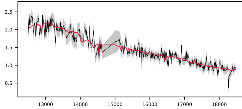
-621287844480163550, 7.3' S/N 13, LSF 22 Å, GALAXY, z = 0.535 , \Delta\chi^2=0 , \chi^2_r=0.6
