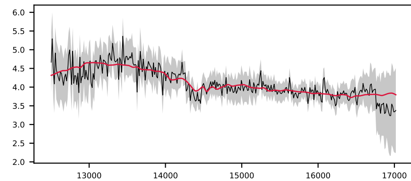
-622047418479360832, 4.8' S/N 33, LSF 29 Å, GALAXY, z = 0.282 , \Delta\chi^2=6 , \chi^2_r=0.2
