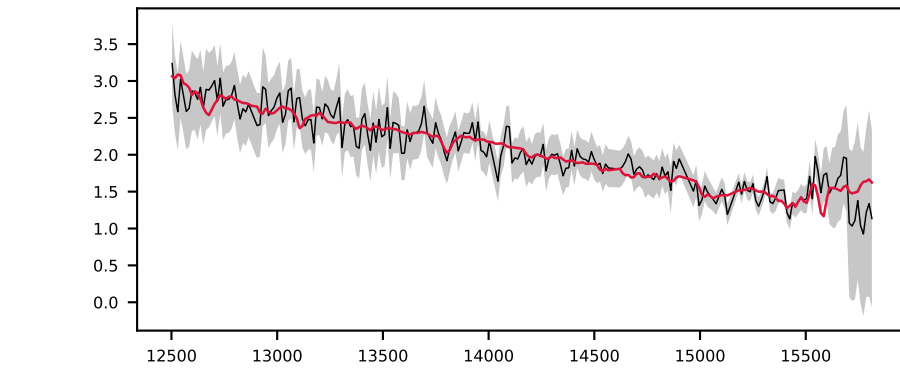
-623393776479001715, 9.6' S/N 13, LSF 13 Å, GALAXY, z = 0.373 , \Delta\chi^2=1 , \chi^2_r=0.3
