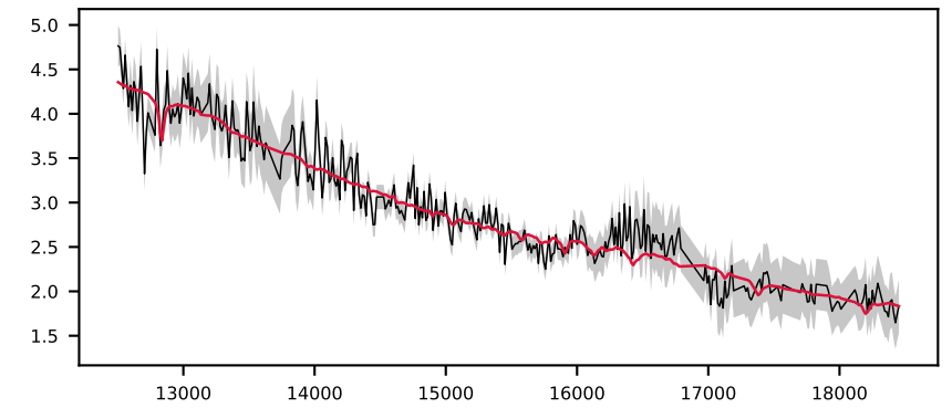
-621007276479388291, 2.5' S/N 22, LSF 20 Å, GALAXY, z = 0.081 , \Delta\chi^2=13 , \chi^2_{\text{r}}=1.0
