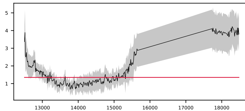
-623426820478910969, 9.7' S/N 20, LSF 13 Å, GALAXY, z = 0.199 , \Delta\chi^2=5 , \chi^2_r=0.5
