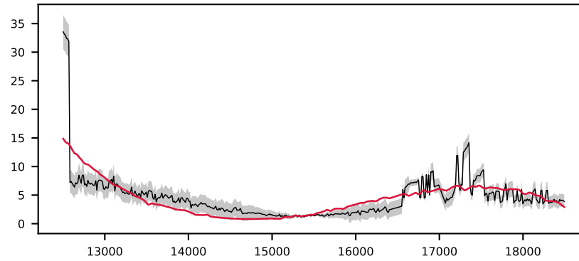
-619621411478546948, 6.1' S/N 32, LSF 46 Å, GALAXY, z = 0.164 , \Delta\chi^2=9 , \chi^2_r=0.5
