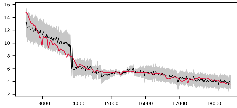
-620884712479294562, 2.0' S/N 46, LSF 14 Å, GALAXY, z = 0.035 , \Delta\chi^2=34 , \chi^2_r=0.7
