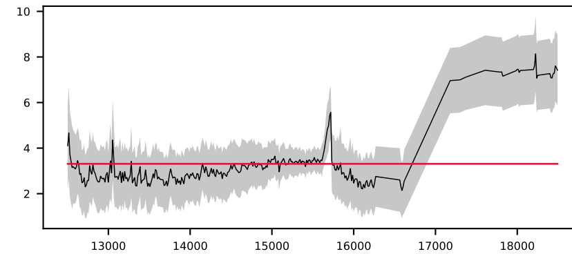
-621512808479085560, 2.2' S/N 24, LSF 12 Å, GALAXY, z = 0.145 , \Delta\chi^2=1 , \chi^2_r=0.1
