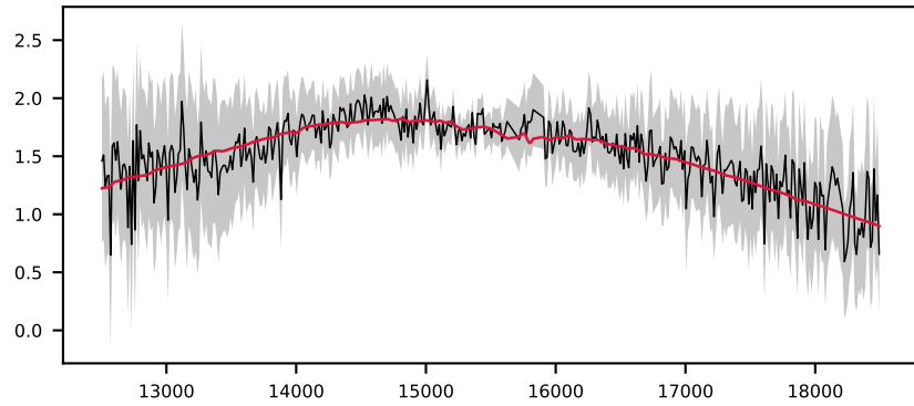
-619243512478837864, 7.1' S/N 13, LSF 34 Å, GALAXY, z = 0.437 , \Delta\chi^2=1 , \chi^2_r=0.6
