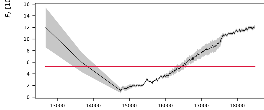
-623448135478896456, 9.8' S/N 45, LSF 26 Å, GALAXY, z = 0.581 , \Delta\chi^2=6 , \chi^2_r=0.6
