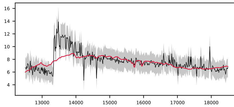
-621421800478751597, 2.1' S/N 47, LSF 15 Å, GALAXY, z = 0.519 , \Delta\chi^2=13 , \chi^2_r=0.2
