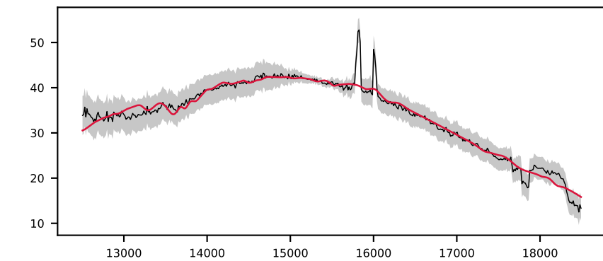
-621441904479032743, 1.8' S/N 107, LSF 40 Å, GALAXY, z = 0.211 , \Delta\chi^2=8 , \chi^2_r=0.4
