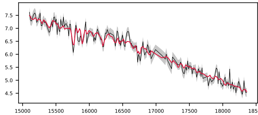
-621196866479263004, 1.9' S/N 39, LSF 19 Å, GALAXY, z = 0.054 , \Delta\chi^2=34 , \chi^2_r=1.7
