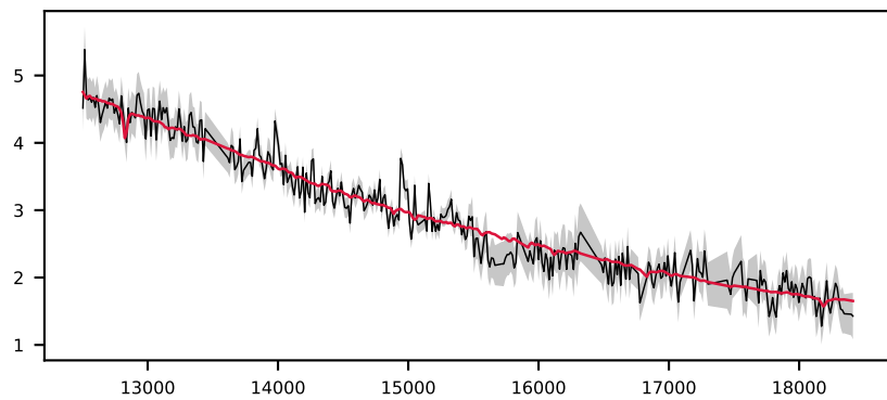
-621124269479306302, 2.1' S/N 21, LSF 19 Å, GALAXY, z = 0.033 , \Delta\chi^2=28 , \chi^2_r=0.8
