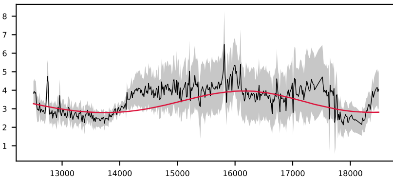
-621645289479075716, 2.7' S/N 24, LSF 37 Å, GALAXY, z = 0.282 , \Delta\chi^2=5 , \chi^2_r=0.2
