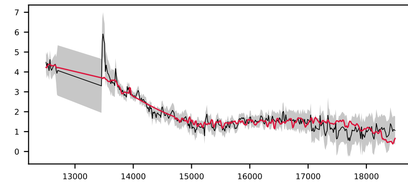
-620984922478553682, 2.5' S/N 16, LSF 9 Å, GALAXY, z = 0.103 , \Delta\chi^2=1113 , \chi^2_r=2.0
