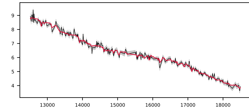
-620941643478211119, 4.6' S/N 43, LSF 13 Å, GALAXY, z = 0.346 , \Delta\chi^2=20 , \chi^2_r=0.5
