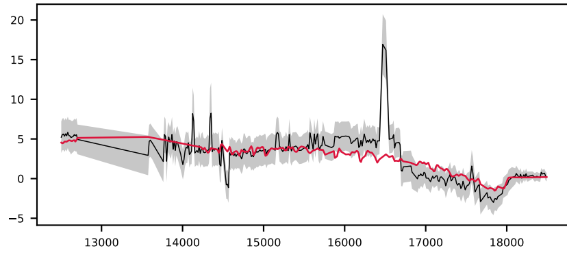
-620469356479209556, 2.6' S/N 21, LSF 13 Å, GALAXY, z = 0.147 , \Delta\chi^2=0 , \chi^2_r=0.1
