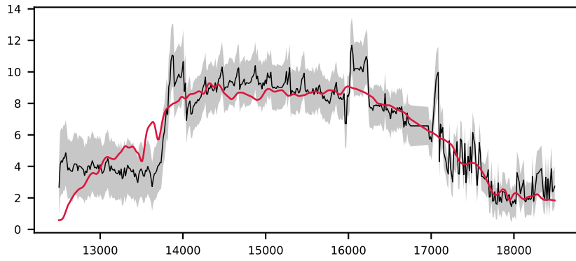
-623448135478896456, 9.8' S/N 45, LSF 26 Å, GALAXY, z = 0.581 , \Delta\chi^2=6 , \chi^2_r=0.6
