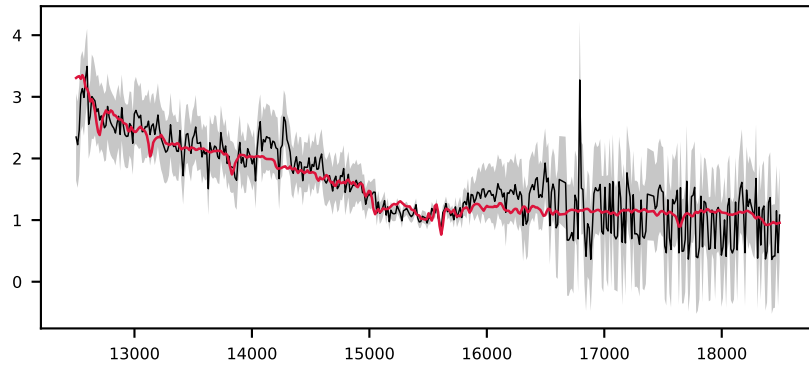
-620877486479742302, 4.7' S/N 15, LSF 15 Å, GALAXY, z = 0.199 , \Delta\chi^2=0 , \chi^2_{\text{r}}=0.3
