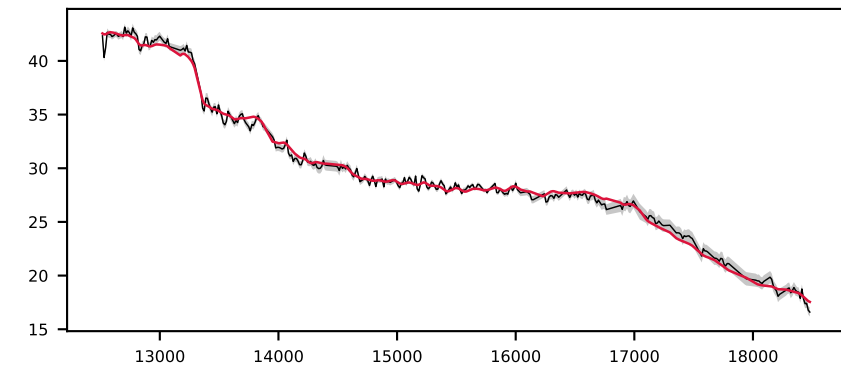
-621385406479043982, 1.6' S/N 129, LSF 53 Å, GALAXY, z = 0.494 , \Delta\chi^2=6 , \chi^2_r=0.7
