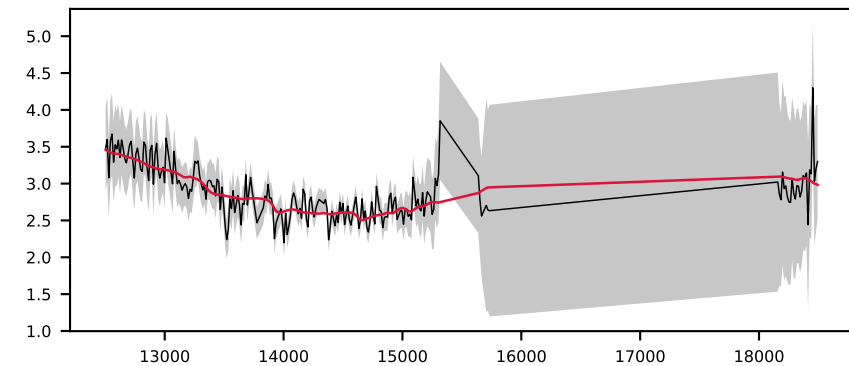
-619279385479497735, 7.6' S/N 18, LSF 12 Å, GALAXY, z = 0.327 , \Delta\chi^2=2 , \chi^2_r=0.1
