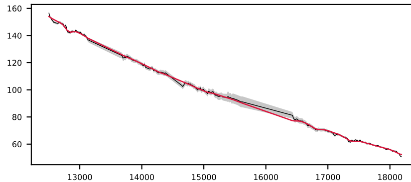
-620997306479135399, 1.0' S/N 227, LSF 31 Å, GALAXY, z = 0.208 , \Delta\chi^2=1876 , \chi^2_r=163.0 X unfittable
