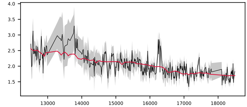
-620657286478590672, 2.7' S/N 13, LSF 20 Å, GALAXY, z = 0.150 , \Delta\chi^2=0 , \chi^2_r=0.2
