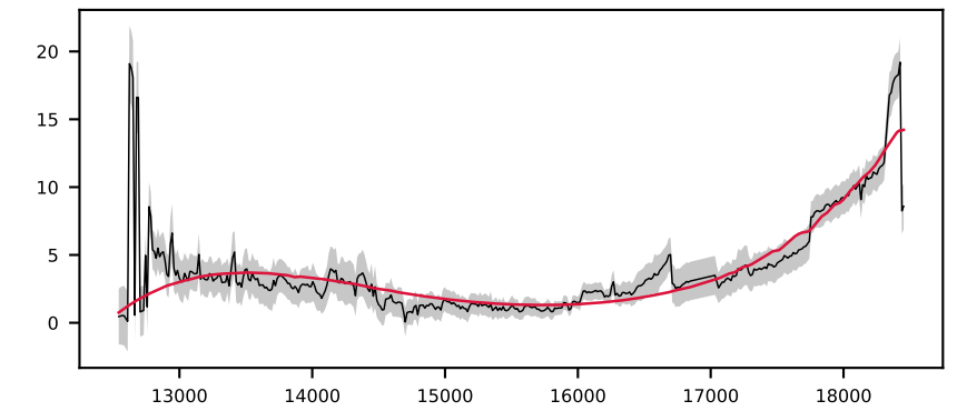
-620154170477930983, 7.1' S/N 22, LSF 13 Å, GALAXY, z = 0.455 , \Delta\chi^2=20 , \chi^2_{\text{r}}=0.5
