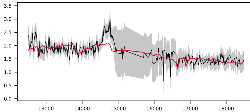
-621429506479476855, 3.5' S/N 15, LSF 18 Å, GALAXY, z = 0.949 , \Delta\chi^2=2 , \chi^2_{\text{r}}=0.5
