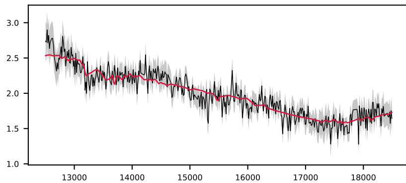
-619416651479155412, 6.5' S/N 19, LSF 20 Å, GALAXY, z = 0.207 , \Delta\chi^2=0 , \chi^2_r=0.6
