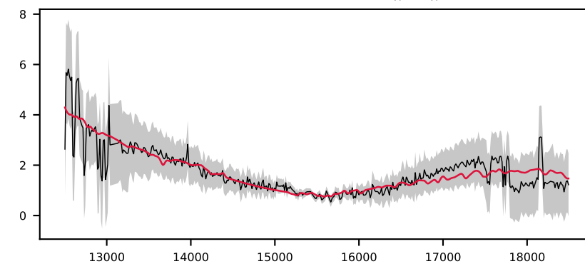
-623281675478760392, 9.2' S/N 13, LSF 17 Å, GALAXY, z = 0.194 , \Delta\chi^2=1 , \chi^2_r=0.2
