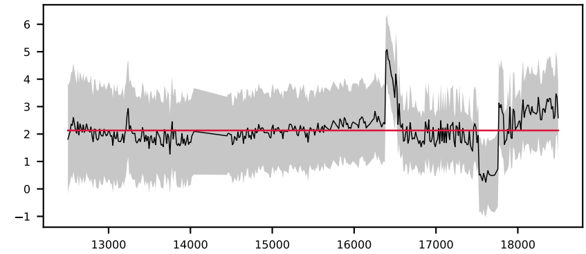
-620297922478361147, 4.6' S/N 15, LSF 17 Å, GALAXY, z = 0.104 , \Delta\chi^2=5 , \chi^2_r=0.3
