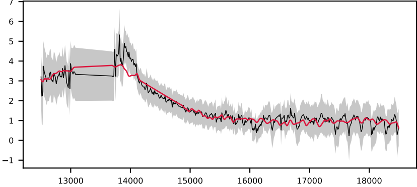
-620238942479862520, 6.2' S/N 12, LSF 16 Å, GALAXY, v = +0 \text{ km/s} , \Delta\chi^2=0 , \chi^2_r=1.5
