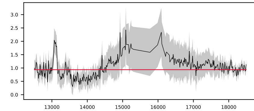
-620876882478315611, 4.0' S/N 12, LSF 13 Å, GALAXY, z = 0.189 , \Delta\chi^2=2 , \chi^2_r=0.4
