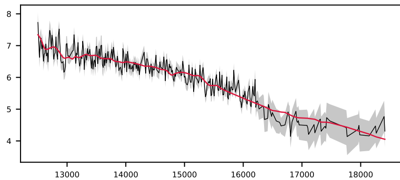
-620273634479174642, 3.2' S/N 28, LSF 44 Å, GALAXY, z = 0.153 , \Delta\chi^2=1 , \chi^2_r=1.1
