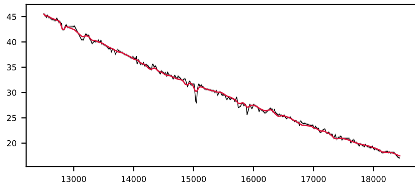
-622942568479360603, 8.1' S/N 133, LSF 16 Å, GALAXY, z = 0.102 , \Delta\chi^2=7 , \chi^2_r=2.0
