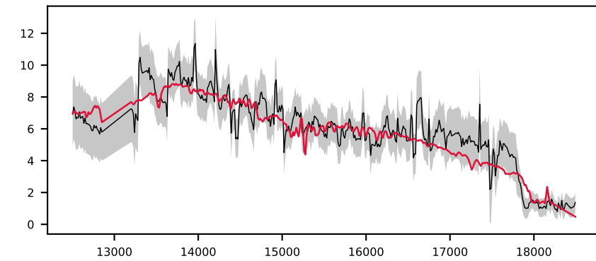
-621892263478034862, 6.6' S/N 42, LSF 11 Å, GALAXY, z = 0.175 , \Delta\chi^2=3 , \chi^2_r=0.3
