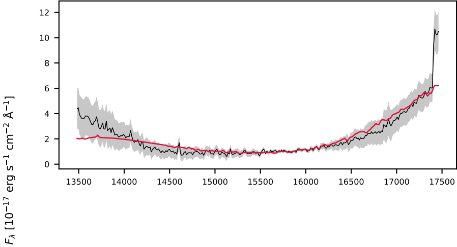
-620871857478608697, 2.2' S/N 12, LSF 15 Å, GALAXY, v = +4839 \text{ km/s} , \Delta\chi^2=9 , \chi^2_r=0.4
