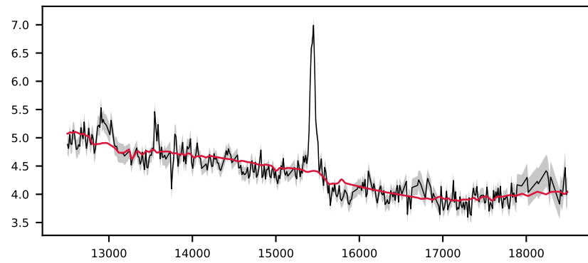
-620588345478662407, 2.5' S/N 30, LSF 19 Å, GALAXY, z = 0.122 , \Delta\chi^2=1 , \chi^2_r=0.6
