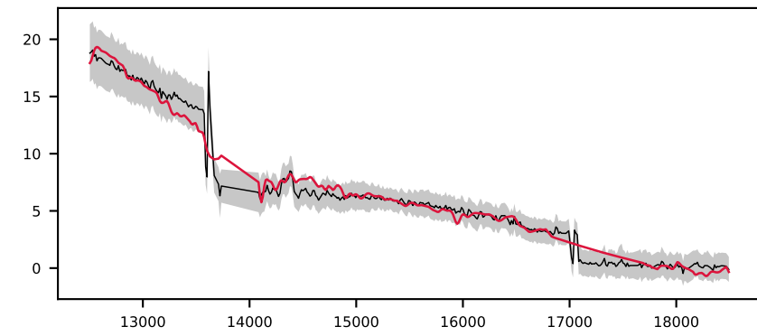
-620555987479189787, 2.2' S/N 45, LSF 15 Å, GALAXY, z = 0.501 , \Delta\chi^2=2 , \chi^2_r=0.2
