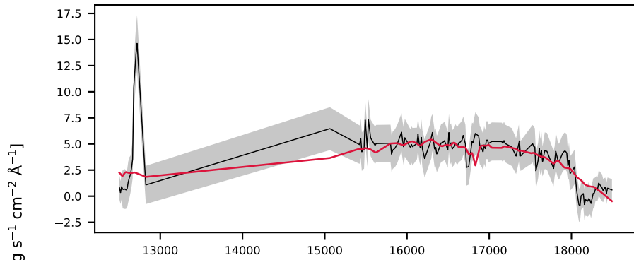
-621383861480135586, 7.2' S/N 19, LSF 37 Å, GALAXY, z = 0.170 , \Delta\chi^2=0 , \chi^2_r=0.0
