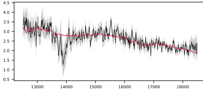
-621117798478245165, 4.4' S/N 15, LSF 20 Å, GALAXY, z = 0.208 , \Delta\chi^2=5 , \chi^2_r=0.3
