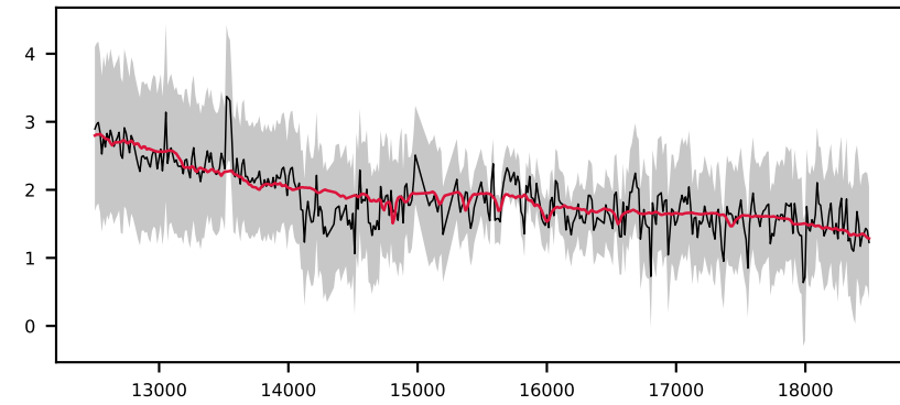
-621264123478590074, 2.5' S/N 19, LSF 25 Å, GALAXY, z = 0.100 , \Delta\chi^2=8 , \chi^2_r=0.7
