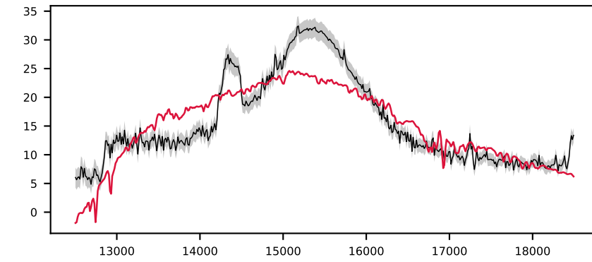
-620626414478709784, 2.2' S/N 87, LSF 12 Å, GALAXY, v = +0 km/s, \Delta\chi^2=0 , \chi^2_r=15.9
