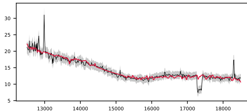
-621130183479214058, 1.5' S/N 107, LSF 11 Å, GALAXY, z = 0.068 , \Delta\chi^2=2 , \chi^2_r=0.6
