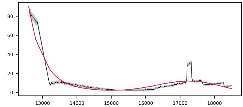
-620682056478696976, 2.1' S/N 51, LSF 13 Å, GALAXY, z = 0.069 , \Delta\chi^2=5848 , \chi^2_r=0.9
