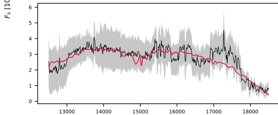
-618622144479050663, 9.6' S/N 22, LSF 26 Å, GALAXY, z = 0.168 , \Delta\chi^2=0 , \chi^2_{\text{r}}=0.0
