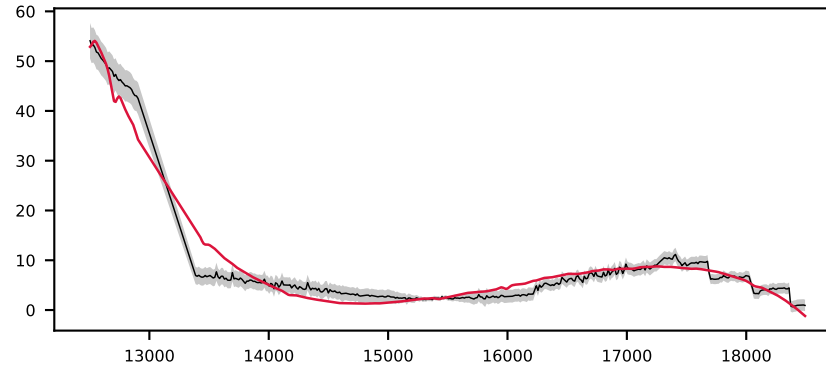
-621182035478647405, 2.1' S/N 38, LSF 16 Å, GALAXY, z = 0.410 , \Delta\chi^2=28 , \chi^2_{\text{r}}=1.9
