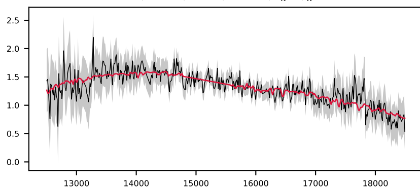
-621623057479032762, 2.5' S/N 13, LSF 14 Å, GALAXY, z = 0.094 , \Delta\chi^2=1 , \chi^2_r=0.3
