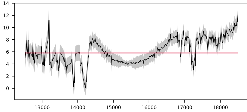
-621194852479246922, 1.8' S/N 47, LSF 18 Å, GALAXY, z = 0.074 , \Delta\chi^2=6 , \chi^2_r=0.6
