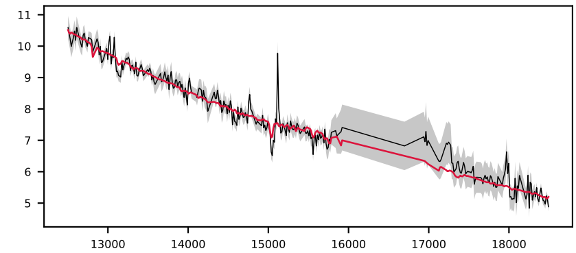
-621477253478649436, 2.7' S/N 49, LSF 14 Å, GALAXY, z = 0.119 , \Delta\chi^2=4 , \chi^2_r=0.3
