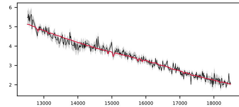
-620444785477761332, 7.6' S/N 30, LSF 21 Å, GALAXY, z = 0.170 , \Delta\chi^2=37 , \chi^2_r=4.5
