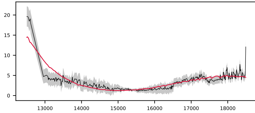
-621659432480063762, 7.1' S/N 26, LSF 36 Å, GALAXY, z = 0.027 , \Delta\chi^2=5 , \chi^2_r=0.9
