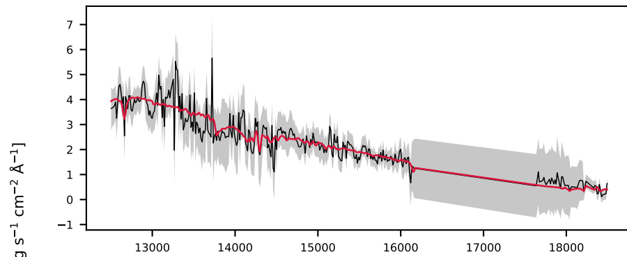
-622708185479829688, 8.6' S/N 17, LSF 16 Å, GALAXY, z = 0.106 , \Delta\chi^2=1 , \chi^2_r=0.6
