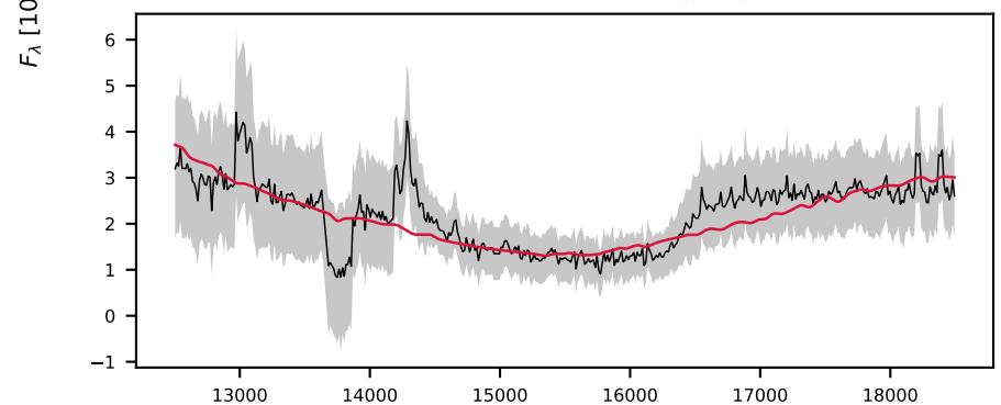
-621572075478806855, 2.5' S/N 21, LSF 18 Å, GALAXY, z = 0.250 , \Delta\chi^2=1 , \chi^2_r=0.4
