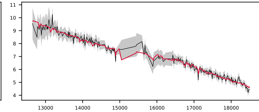
-622025777479386791, 4.8' S/N 54, LSF 16 Å, GALAXY, z = 0.945 , \Delta\chi^2=10 , \chi^2_r=0.3
