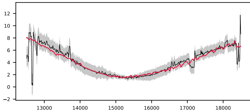
-620404257479078049, 2.5' S/N 34, LSF 29 Å, GALAXY, z = 0.208 , \Delta\chi^2=1 , \chi^2_r=0.7
