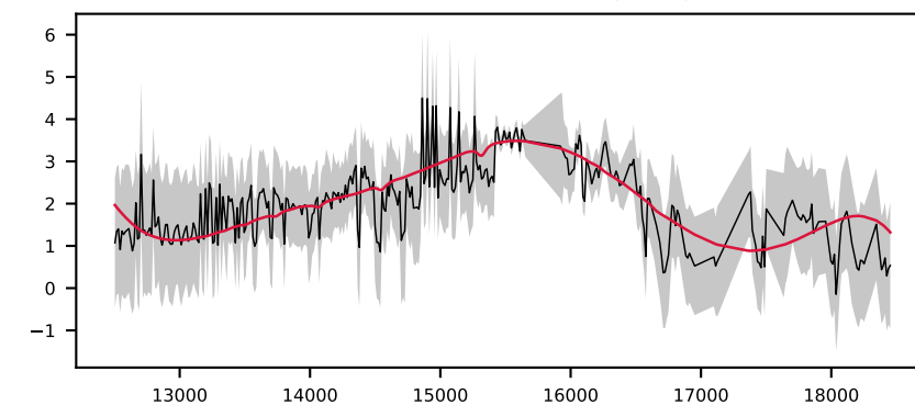
-622120828479092888, 4.5' S/N 13, LSF 12 Å, GALAXY, z = 0.309 , \Delta\chi^2=6 , \chi^2_r=0.7
