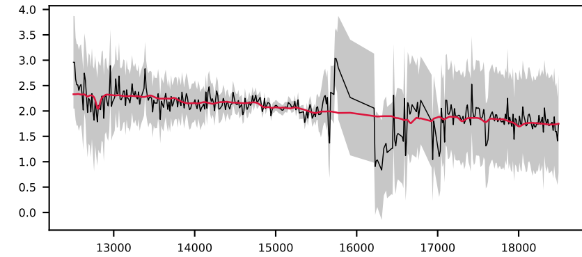
-622166408479069860, 4.7' S/N 20, LSF 32 Å, GALAXY, z = 0.094 , \Delta\chi^2=0 , \chi^2_r=0.4
