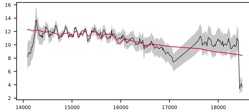
-622202138478876627, 4.8' S/N 62, LSF 24 Å, GALAXY, z = 0.182 , \Delta\chi^2=59 , \chi^2_r=1.1
