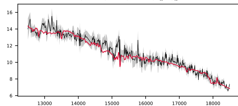
-621447045480055097, 6.7' S/N 74, LSF 12 Å, GALAXY, z = 0.343 , \Delta\chi^2=5 , \chi^2_r=0.8
