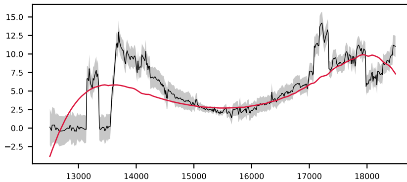
-620691689479288485, 2.3' S/N 40, LSF 13 Å, GALAXY, z = 0.373 , \Delta\chi^2=3 , \chi^2_r=0.7
