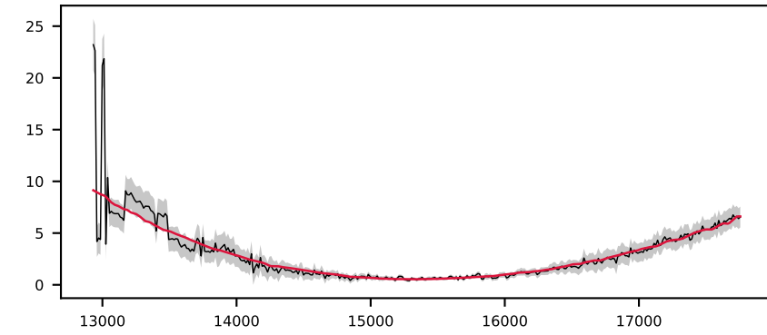
-620136222479351547, 4.2' S/N 16, LSF 32 Å, STAR, v = -600 \text{ km/s} , \Delta\chi^2=\text{inf} , \chi^2_r=0.2
