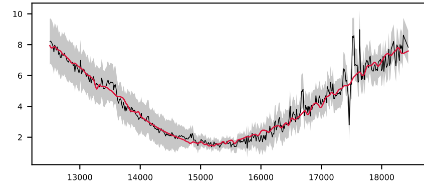
-621465754479115276, 2.0' S/N 38, LSF 15 Å, GALAXY, z = 0.030 , \Delta\chi^2=24 , \chi^2_{\text{r}}=0.4
