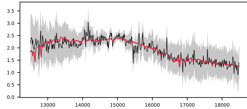
-622959768479141834, 7.9' S/N 18, LSF 26 Å, GALAXY, z = 0.057 , \Delta\chi^2=3 , \chi^2_r=0.7
