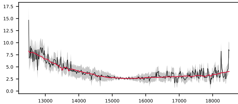
-621411933479158532, 2.0' S/N 31, LSF 22 Å, GALAXY, z = 0.581 , \Delta\chi^2=2 , \chi^2_r=0.3
