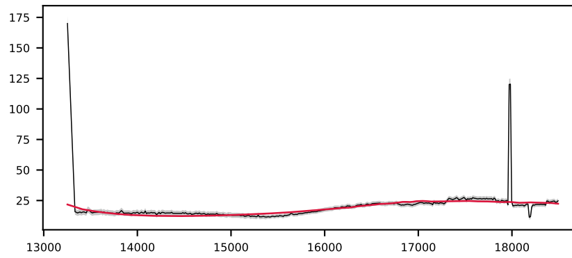
-621302672478727323, 1.9' S/N 90, LSF 14 Å, GALAXY, z = 0.029 , \Delta\chi^2=34 , \chi^2_r=1.0
