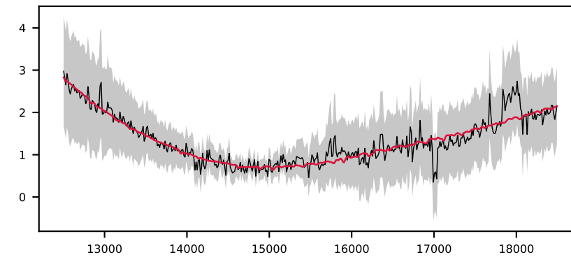
-622228846478928760, 4.9' S/N 14, LSF 52 Å, GALAXY, z = 0.886 , \Delta\chi^2=3 , \chi^2_{\text{r}}=1.1
