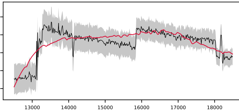
-621182035478647405, 2.1' S/N 38, LSF 16 Å, GALAXY, z = 0.410 , \Delta\chi^2=28 , \chi^2_{\text{r}}=1.9
