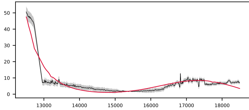
-620638518479241561, 2.2' S/N 39, LSF 14 Å, GALAXY, z = 0.240 , \Delta\chi^2=5 , \chi^2_{\text{r}}=0.3
