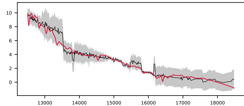
-623095009478753751, 8.5' S/N 27, LSF 14 Å, GALAXY, z = 0.090 , \Delta\chi^2=6 , \chi^2_r=0.4
