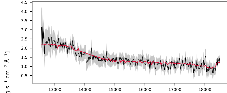
-622949937479118949, 7.9' S/N 12, LSF 12 Å, GALAXY, z = 0.050 , \Delta\chi^2=10 , \chi^2_r=0.7
