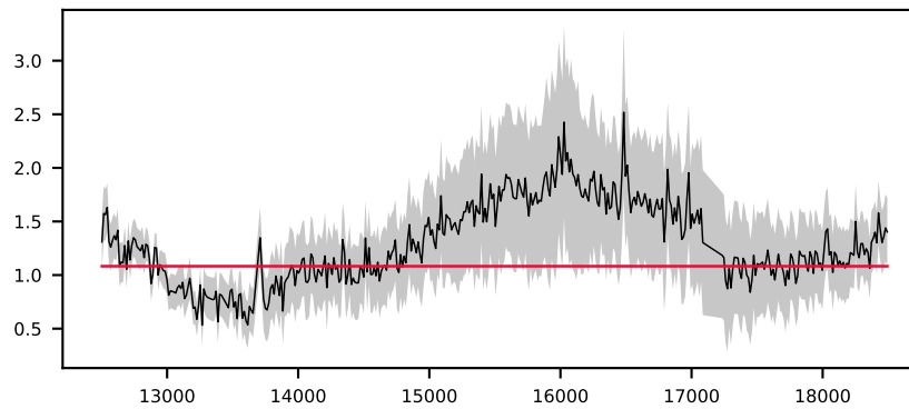
-620585686479305940, 2.6' S/N 14, LSF 16 Å, GALAXY, z = 0.172 , \Delta\chi^2=11 , \chi^2_{\text{r}}=0.5
