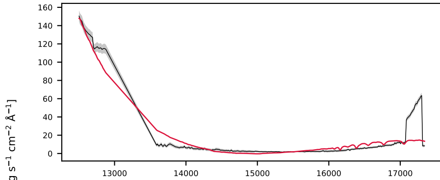
-621159739479275964, 1.9' S/N 31, LSF 16 Å, GALAXY, z = 0.054 , \Delta\chi^2=21 , \chi^2_r=2.0
