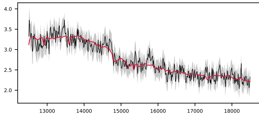
-620700570478676743, 2.1' S/N 22, LSF 18 Å, GALAXY, z = 0.089 , \Delta\chi^2=4 , \chi^2_r=4.0
