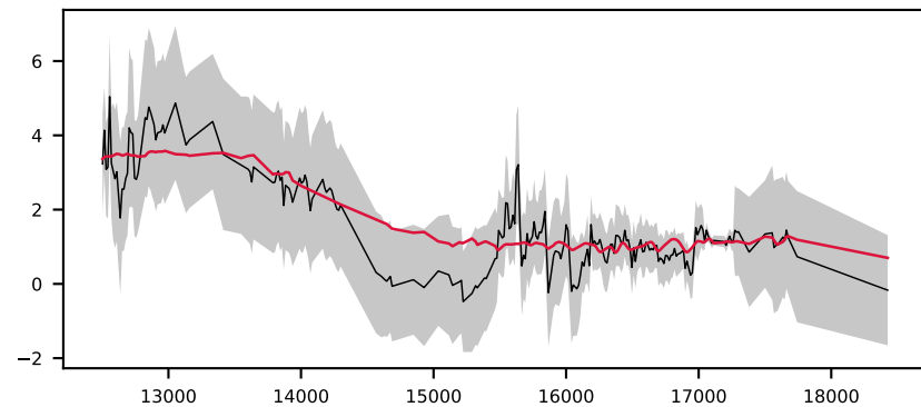
-621022966479633612, 4.0' S/N 12, LSF 20 Å, GALAXY, z = 0.503 , \Delta\chi^2=1 , \chi^2_r=0.2
