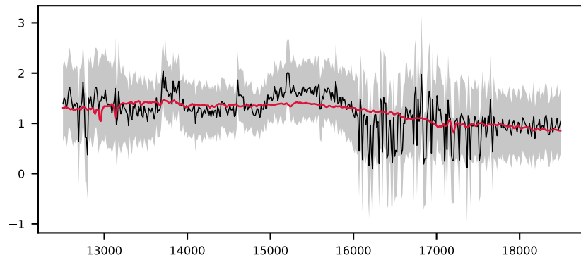
-619334450478229668, 8.1' S/N 13, LSF 9 Å, GALAXY, z = 0.021 , \Delta\chi^2=2 , \chi^2_r=0.3
