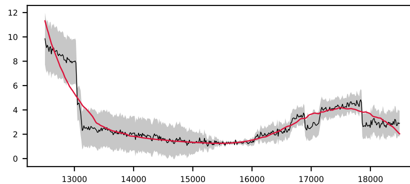
-620589353478628291, 2.6' S/N 21, LSF 15 Å, GALAXY, z = 0.115 , \Delta\chi^2=1 , \chi^2_r=0.1
