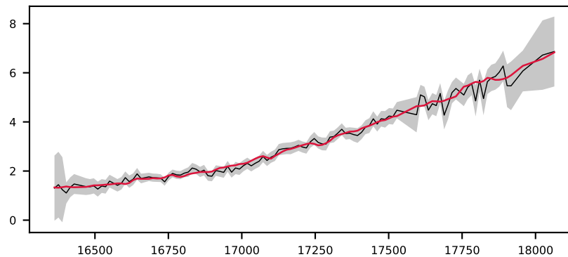
-620547806479591952, 4.2' S/N 22, LSF 40 Å, GALAXY, z = 0.379 , \Delta\chi^2=4 , \chi^2_r=1.2
