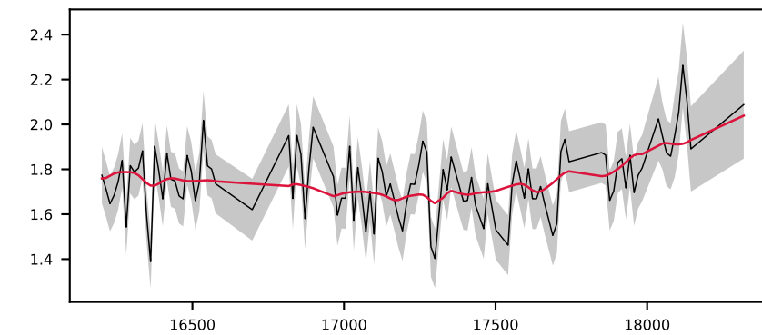
-623087371478616480, 8.6' S/N 14, LSF 19 Å, GALAXY, z = 0.089 , \Delta\chi^2=3 , \chi^2_{\text{r}}=0.9
