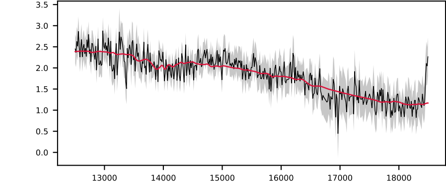
-620871857478608697, 2.2' S/N 12, LSF 15 Å, GALAXY, v = +4839 \text{ km/s} , \Delta\chi^2=9 , \chi^2_r=0.4
