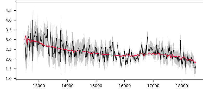
-620617250478001723, 6.0' S/N 16, LSF 13 Å, GALAXY, z = 0.109 , \Delta\chi^2=1 , \chi^2_r=0.8
