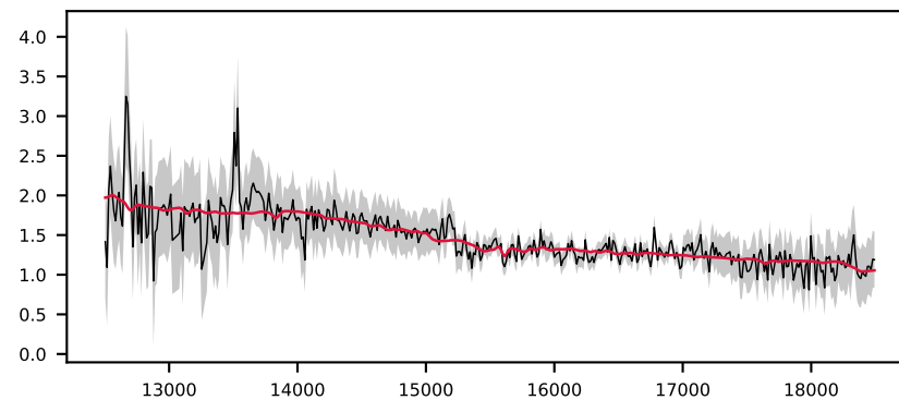
-623201448479309061, 9.1' S/N 12, LSF 12 Å, GALAXY, z = 0.574 , \Delta\chi^2=10 , \chi^2_r=1.1
