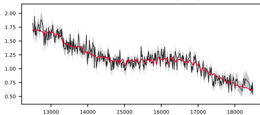
-620514716479755261, 5.1' S/N 13, LSF 20 Å, GALAXY, z = 0.524 , \Delta\chi^2=10 , \chi^2_r=0.6
