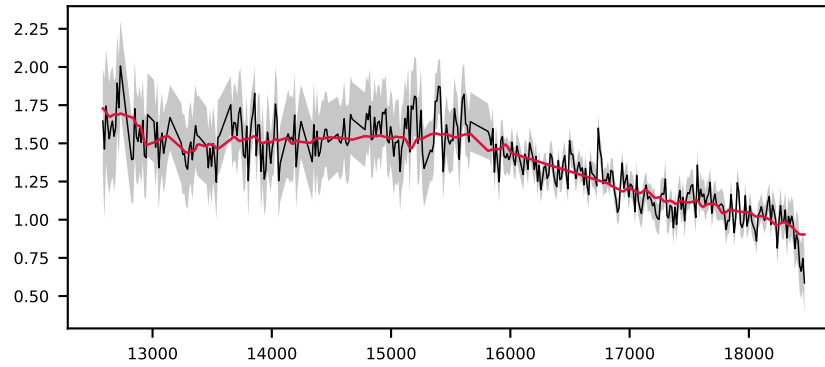
-620753306478644452, 2.2' S/N 13, LSF 14 Å, GALAXY, z = 0.152 , \Delta\chi^2=11 , \chi^2_r=0.5
