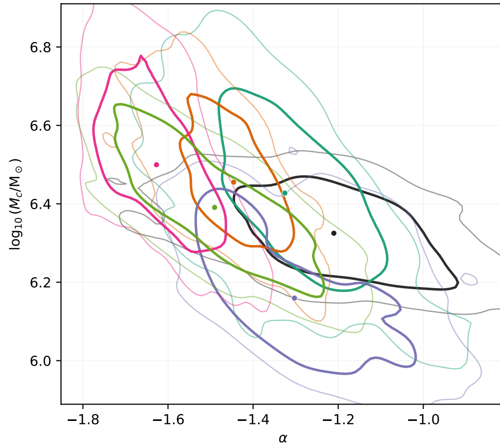
Schechter parameters
