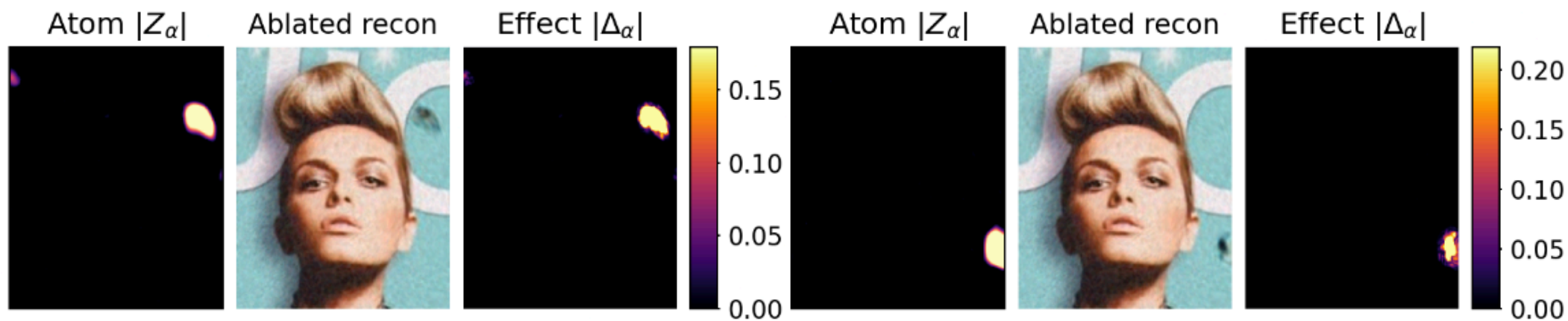
SIREN
