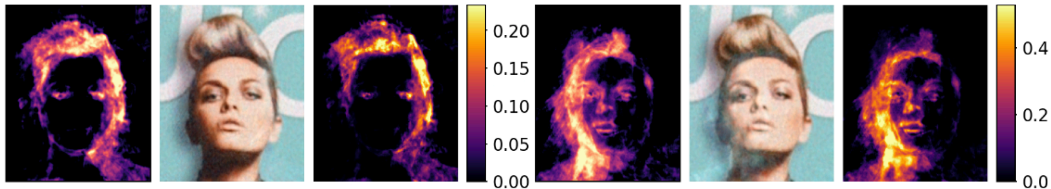
FFMLP
