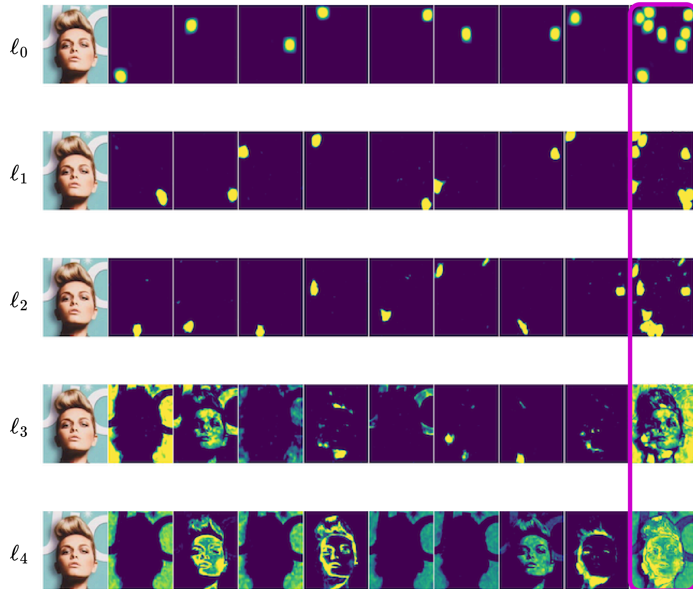
SIREN
