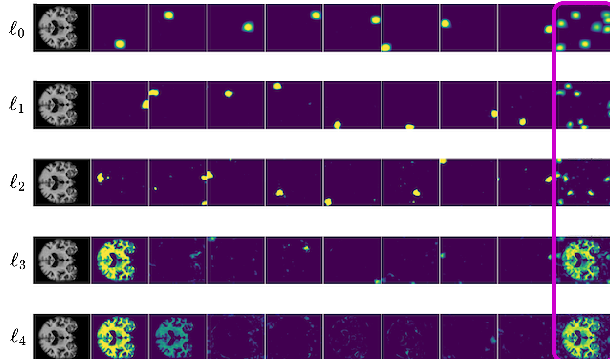
SIREN
