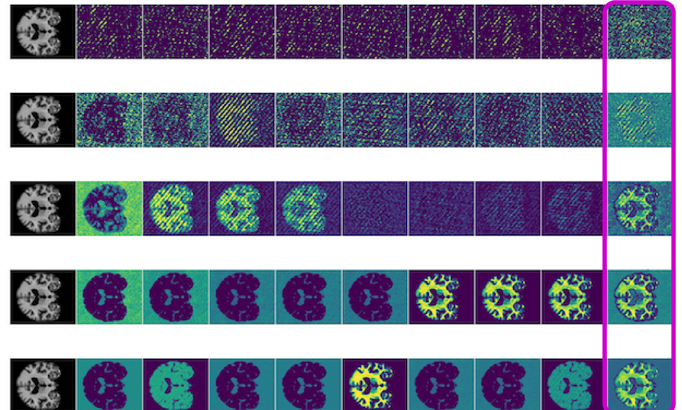
FFMLP
