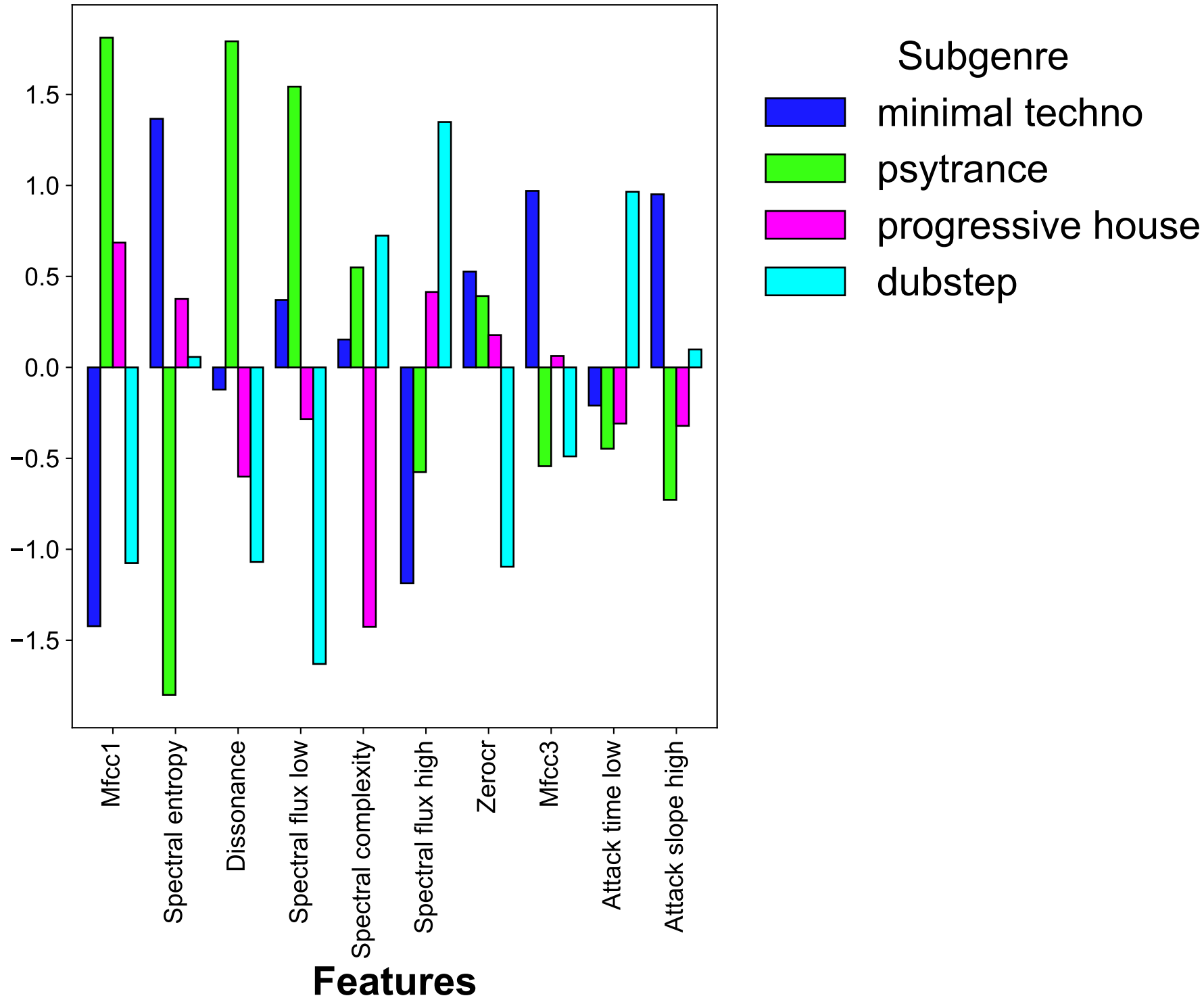
Coefficient values
