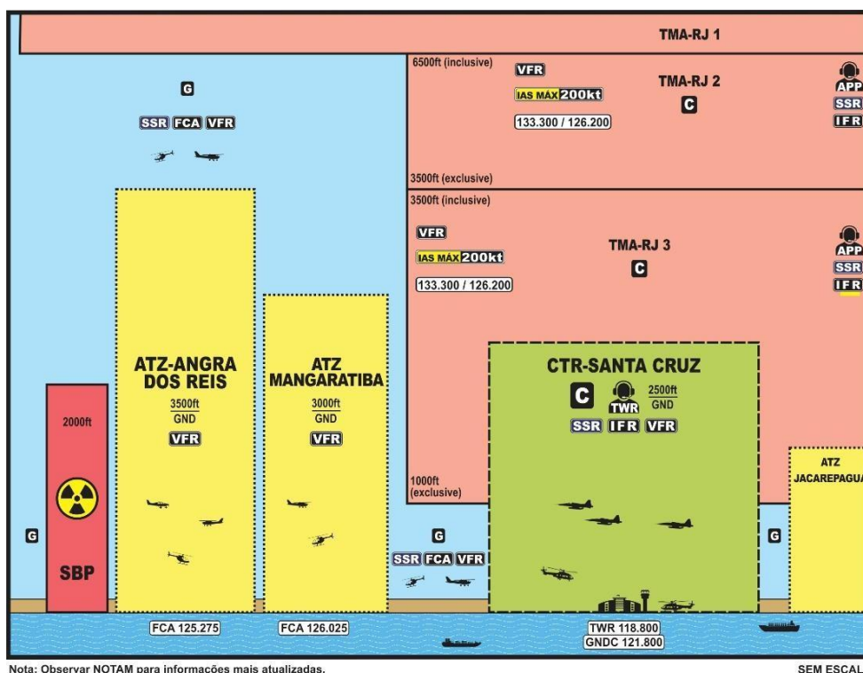
Figura 10 – Vista em Perfil da CTR-SANTA CRUZ, ATZ ANGRA e ATZ-MANGARATIBA
