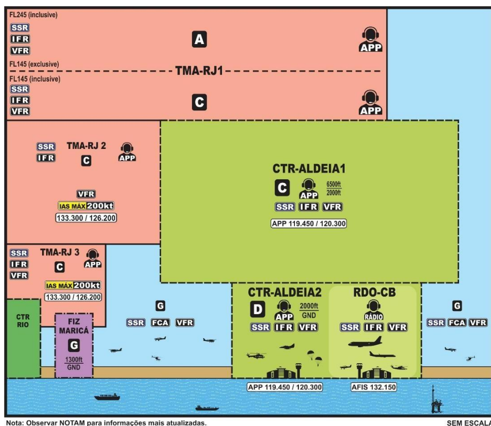
Figura 11 – Vista em Perfil da CTR-ALDEIA
