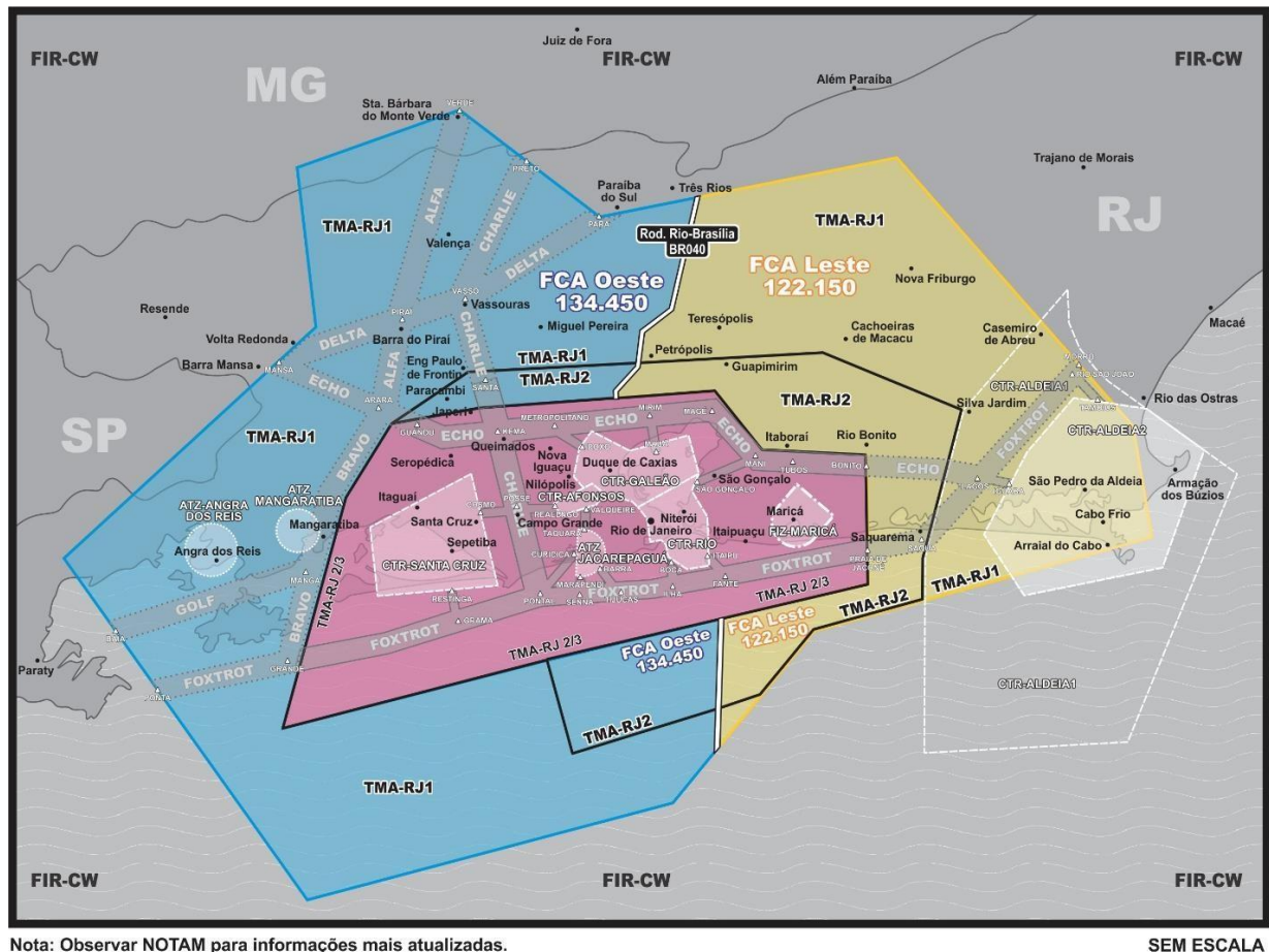
Figura 14- Uso das FCA na TMA-RJ
