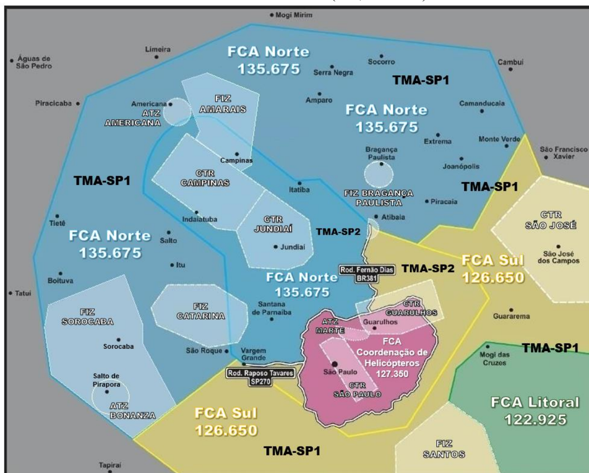
Figura 16 - Uso das FCA para helicópteros
