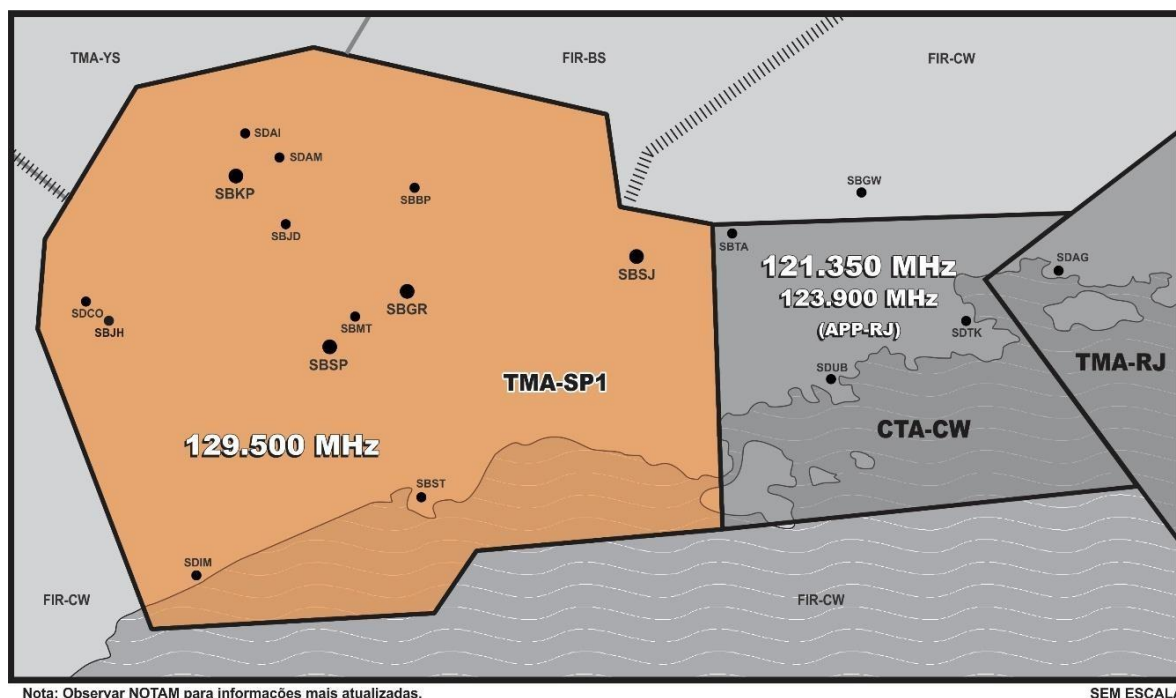
Figura 7- Frequências para prestação do Serviço de Informação de Voo e Alerta
