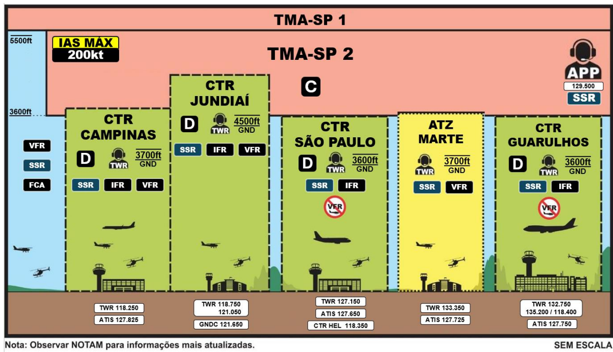
Figura 3 – Vista em Perfil da TMA-SP 2
