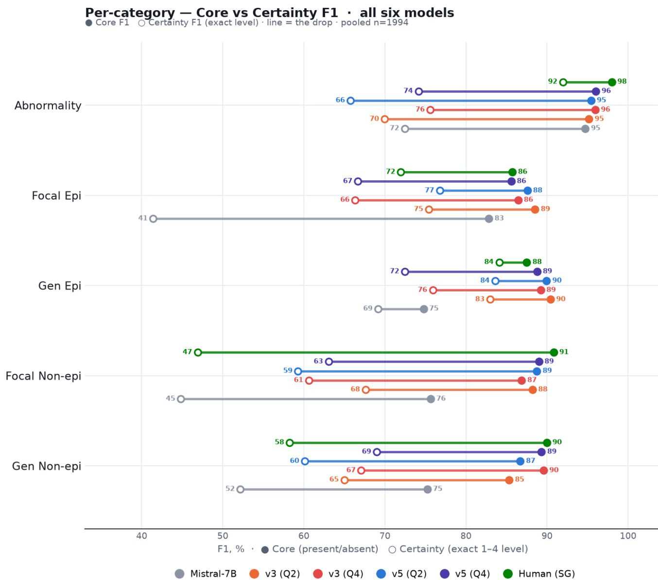
Figure 2: Per-category Core vs Certainty F1
