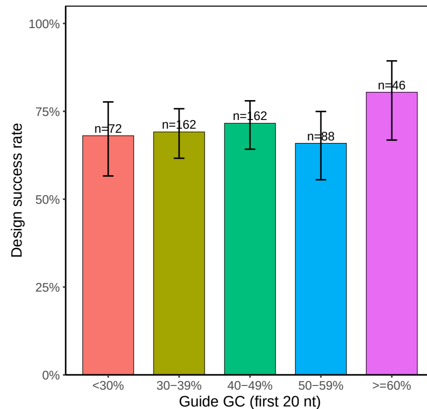
Guide GC, first 20 nt
