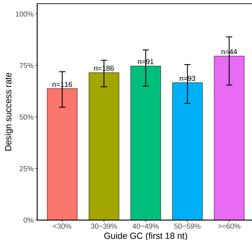
Guide GC, first 18 nt
