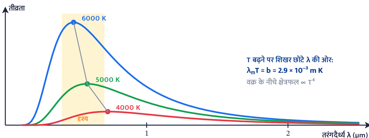
तीन तापों पर कृष्णिका स्पेक्ट्रम – वीन का विस्थापन नियम
