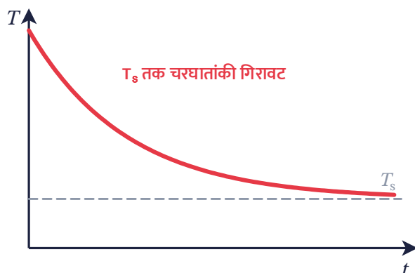
ताप बनाम समय
