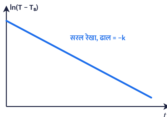
\ln(T - T_s) बनाम समय रैखिक
