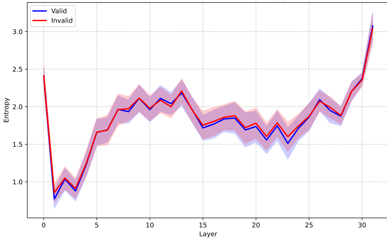
Llama-3.1-8B (Finance, T=1.0) - Entropy
