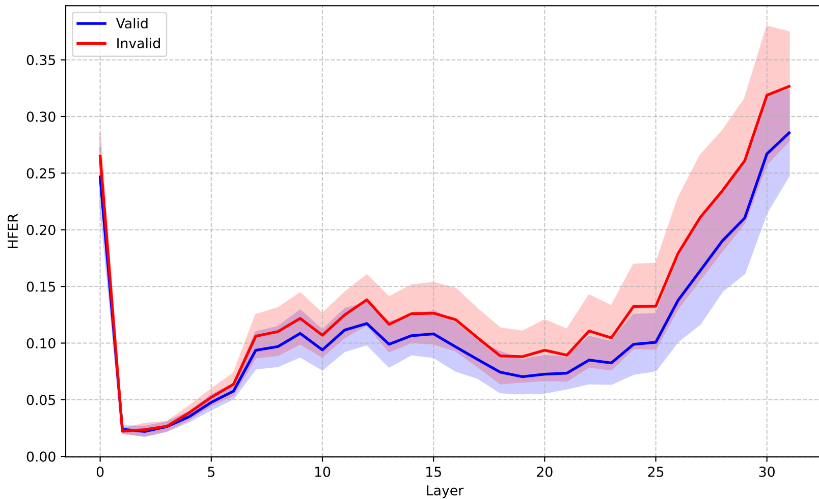
Llama-3.1-8B (General) - HFER
