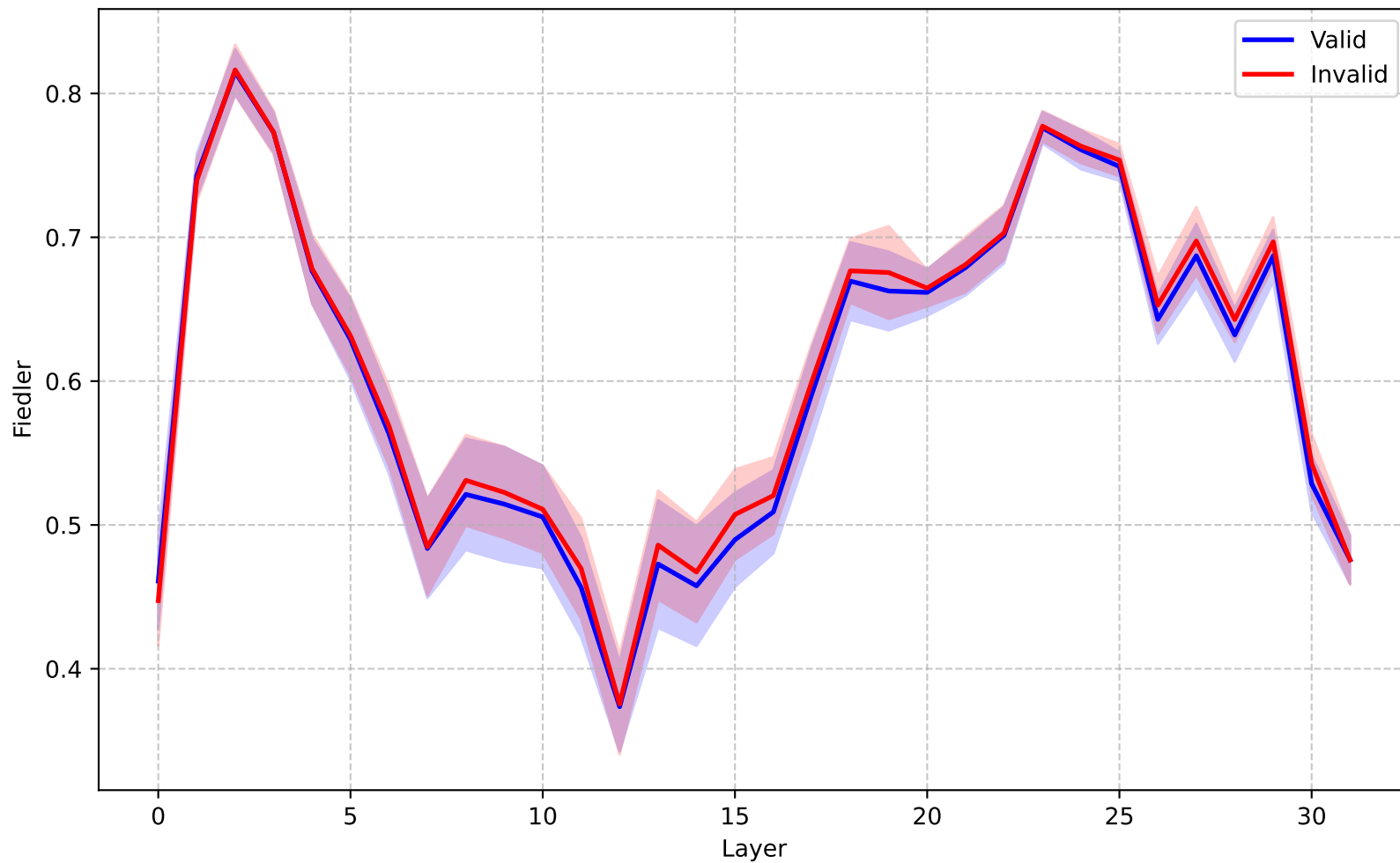
Llama-3.1-8B (Finance, T=1.0) - Fiedler
