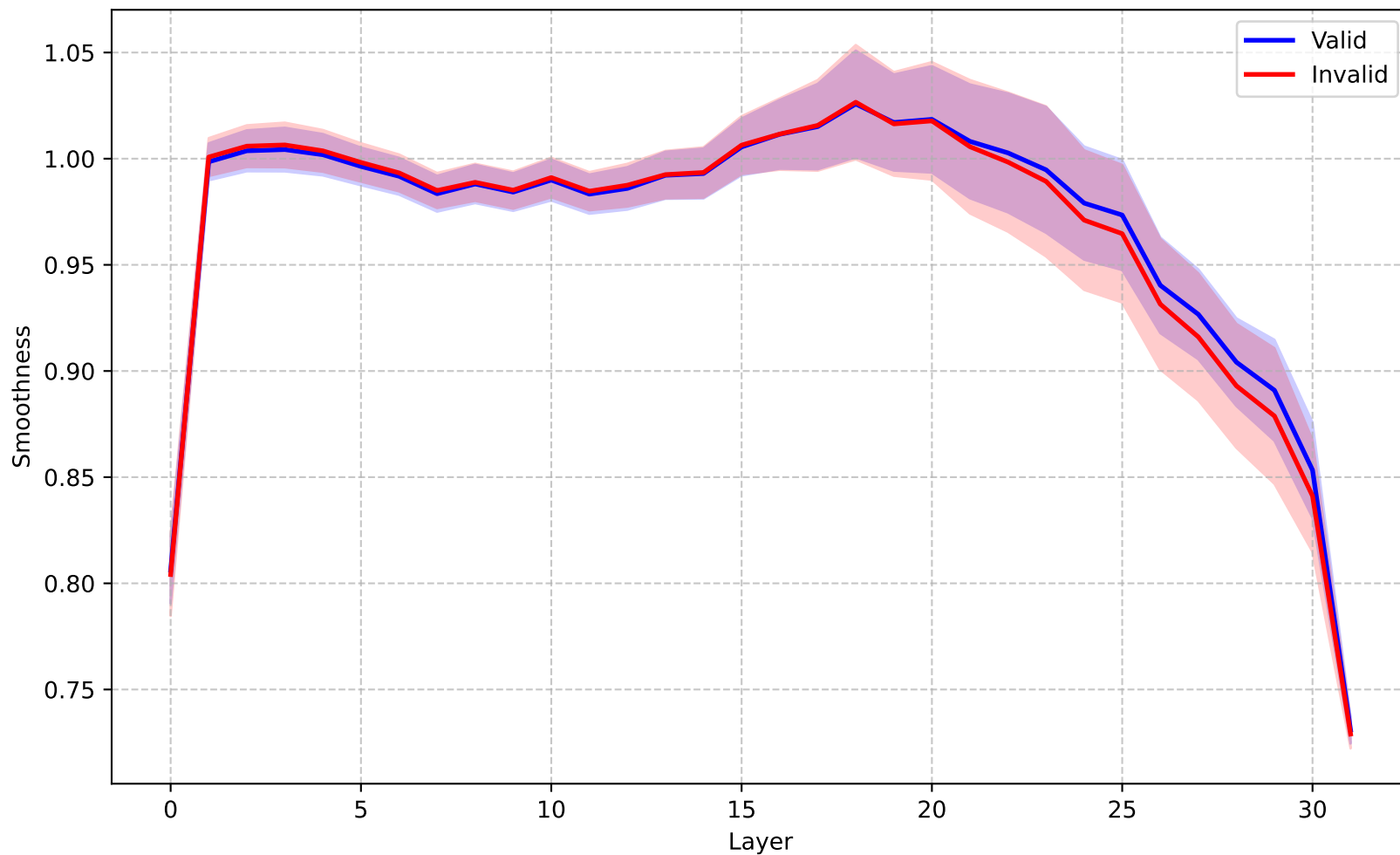
Llama-3.1-8B (Finance, T=1.0) - Smoothness
