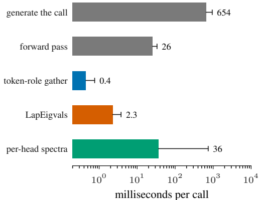
(b) cost per call, Llama-3.2-1B
