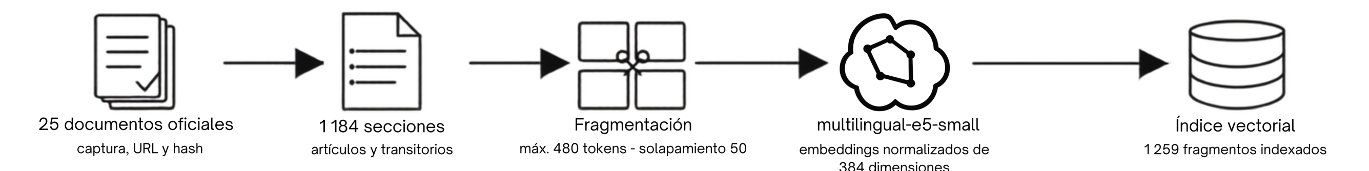
Fig. 1. Indexación reproducible del corpus. Los documentos oficiales se transforman en secciones, fragmentos y representaciones vectoriales normalizadas antes de construir el índice local.
