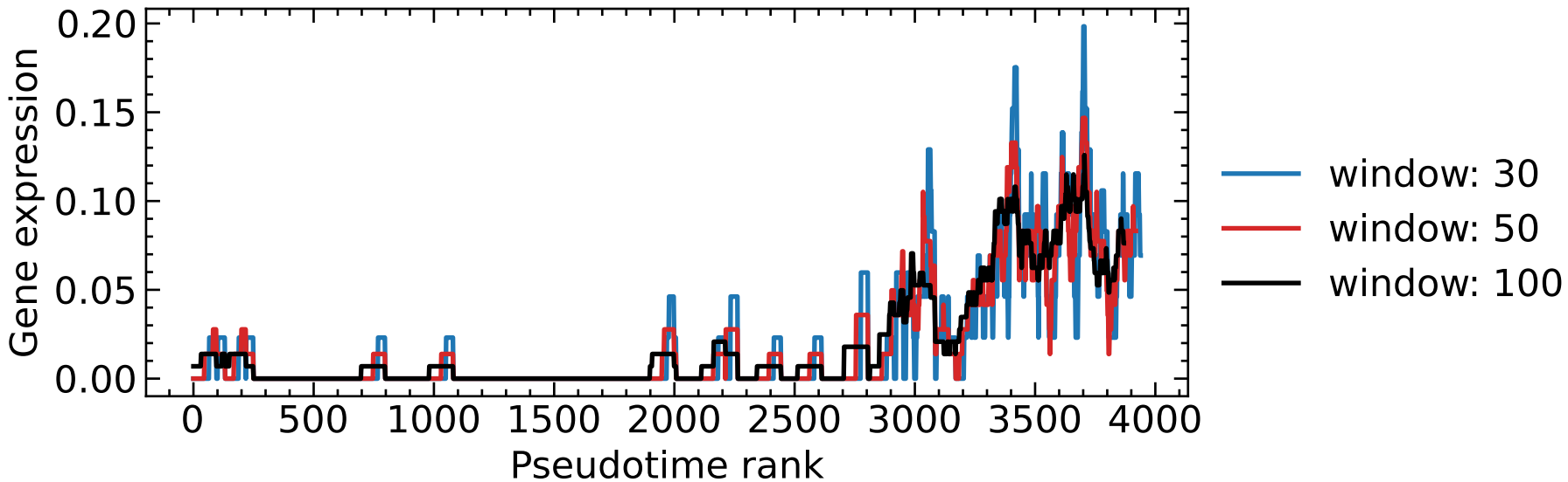
Gene MCOLN2
