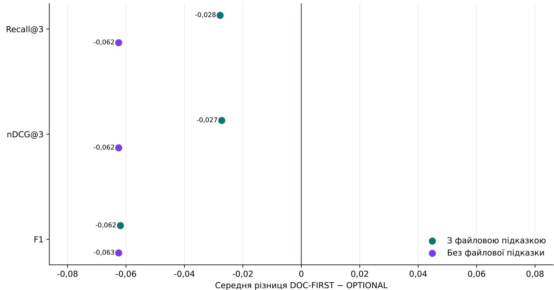
Рисунок 4.3 - Різниця DOC-FIRST проти OPTIONAL за наявності файлової підказки
