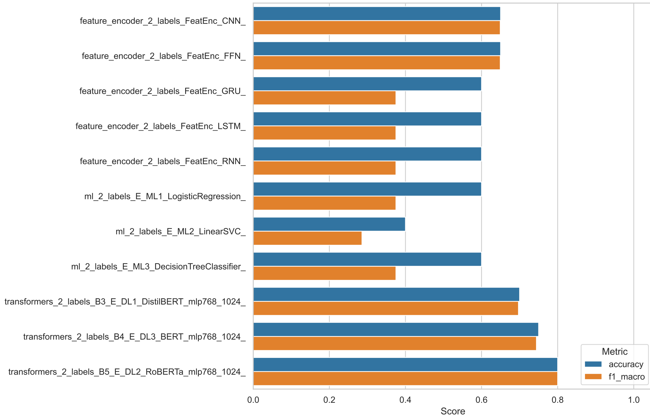
Model Comparison (2-Label) - Accuracy vs F1 Macro
