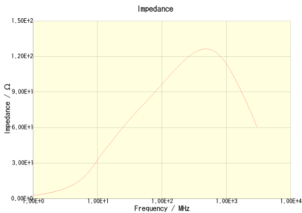
MPZ2012S101AT000
