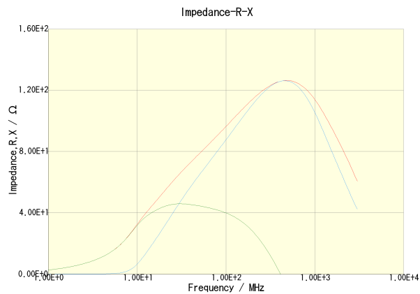
MPZ2012S101AT000(I)MPZ2012S101AT000(R)MPZ2012S101AT000(X)
