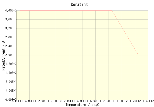
MPZ2012S101AT000
