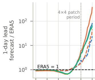
Z500
