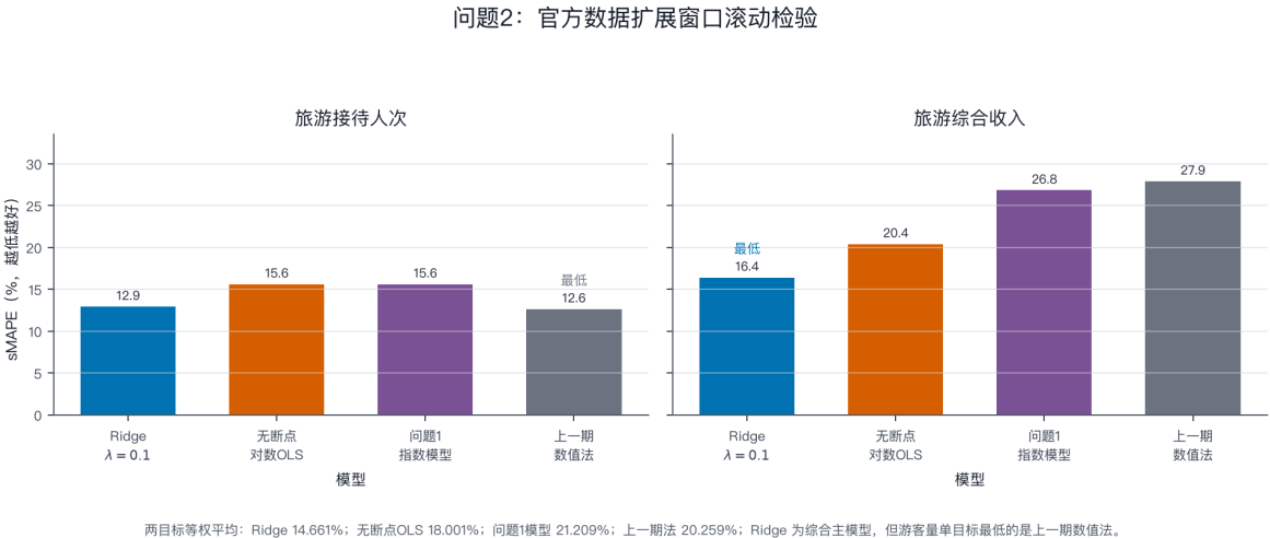
图 2 问题 2 候选模型的时间有序评判
