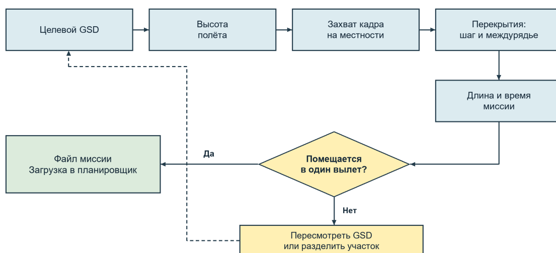
Рисунок 3 — Расчётная цепочка полётного планирования: от целевого GSD к файлу миссии; если миссия не помещается в вылет — пересматриваем GSD или делим участок.
