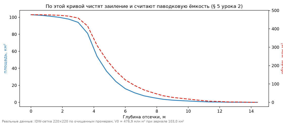
Рис. 3. Кривая «уровень-площадь-объём»: V0 = 476,9 млн м³ при зеркале 103,0 км².
