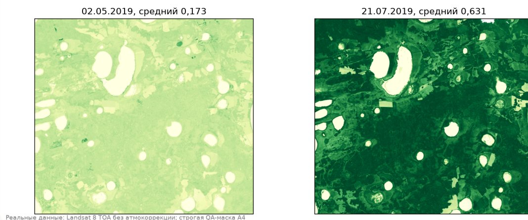
Рис. 4. Поток меняется, запас остаётся: средний NDVI окна 02.05.2019 — 0,173, 21.07.2019 — 0,631 (та же сцена и маска, что в A4/A5).
