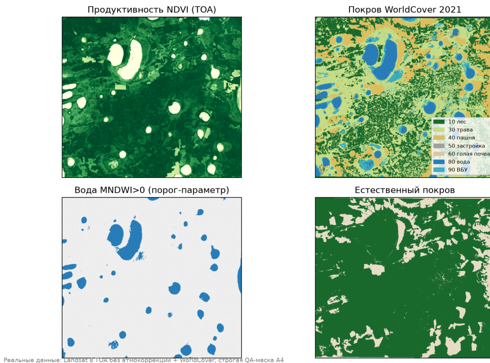
Рис. 3. Витрина индикаторов услуг (таблица §4.1) в одном окне СКО на 21.07.2019: средний NDVI 0,631, вода по MNDWI 7,91 %, естественный покров 83,14 %.
