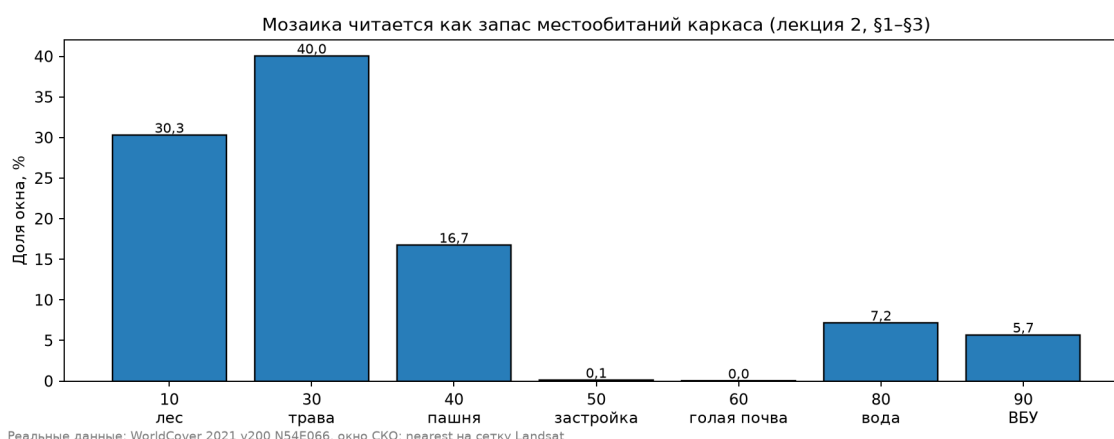
Рис. 4 (Тема 13.3). Мозаика окна СКО: доли WorldCover, Шеннон 1,387
