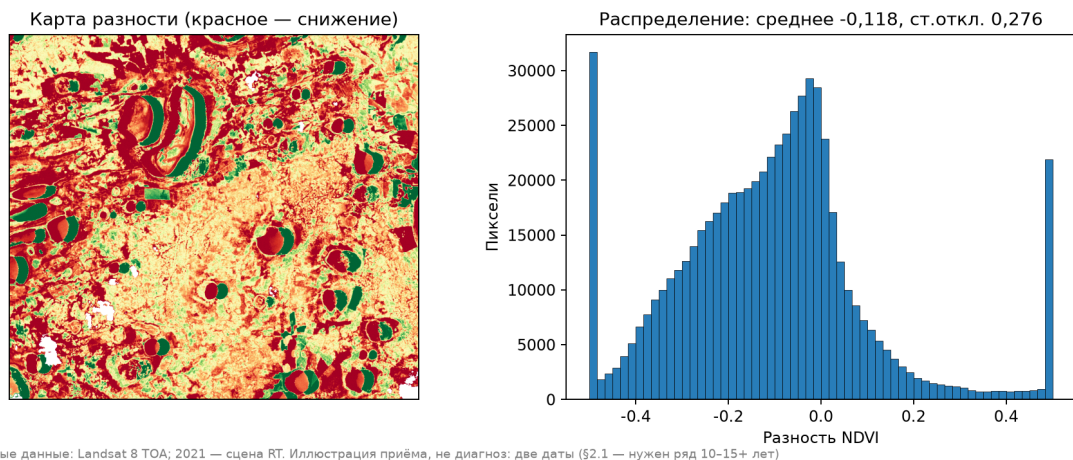
Рис. 5. Разность NDVI 10.07.2021–05.07.2019 (среднее -0,118 , ст.откл. 0,276 ): так выглядит приём «карта очагов» (§4.1) — иллюстрация, не диагноз (две даты).
