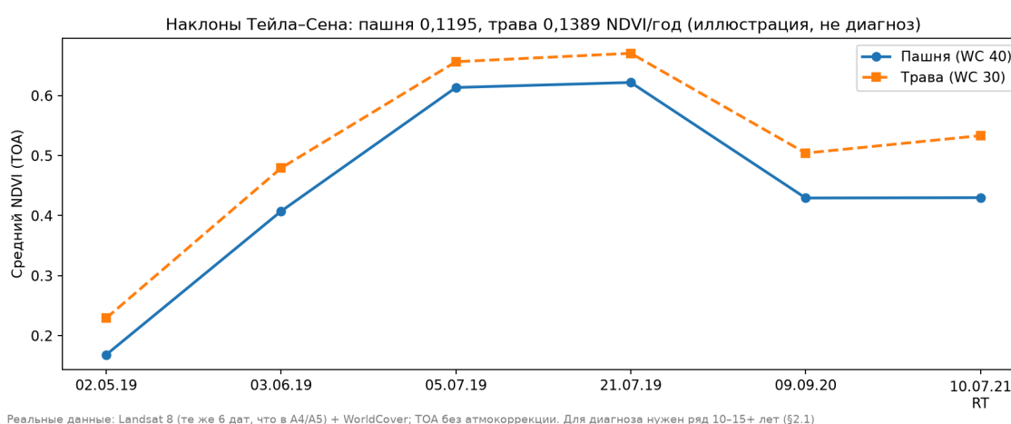
Рис. 3 (Тема 13.3). Иллюстрация метода тренда: NDVI пашни и травы
