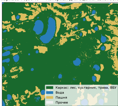
Рис. 3 (Тема 13.2). Каркас окна СКО: зелёная инфраструктура и вода на пашне
