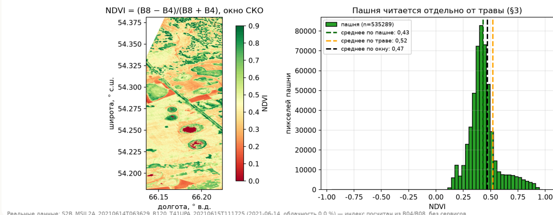
Рисунок 2 — NDVI своими руками: сцена
