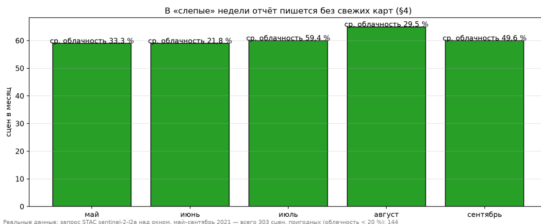
Рис. 2 (Тема ПЗ.2). Что видит сервис: сцены Sentinel-2 за сезон
