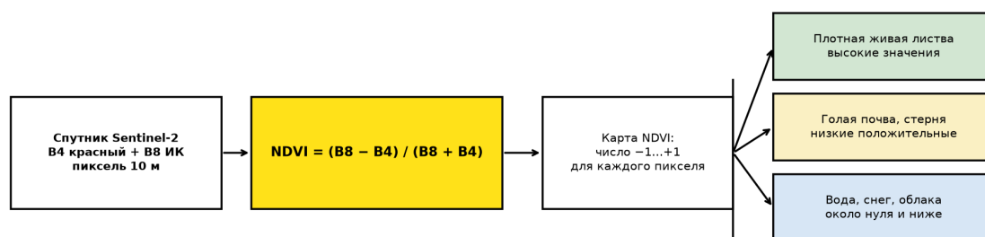
Рис. 1 (Тема ПЗ.1). Путь от спутникового снимка к карте NDVI
