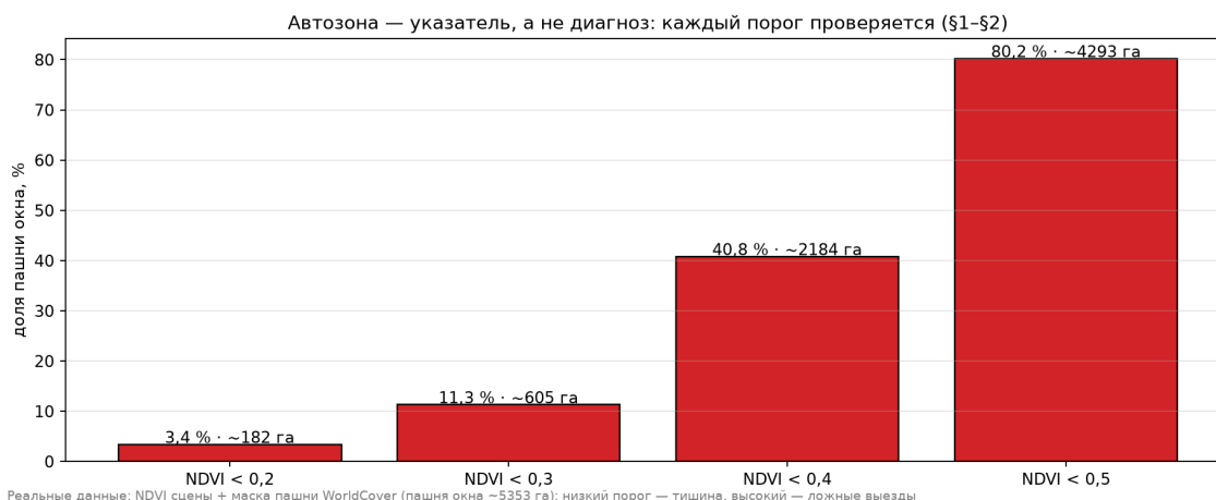
Рис. 2 (Тема П3.3). Порог решает, сколько ехать: пашня ниже порога
