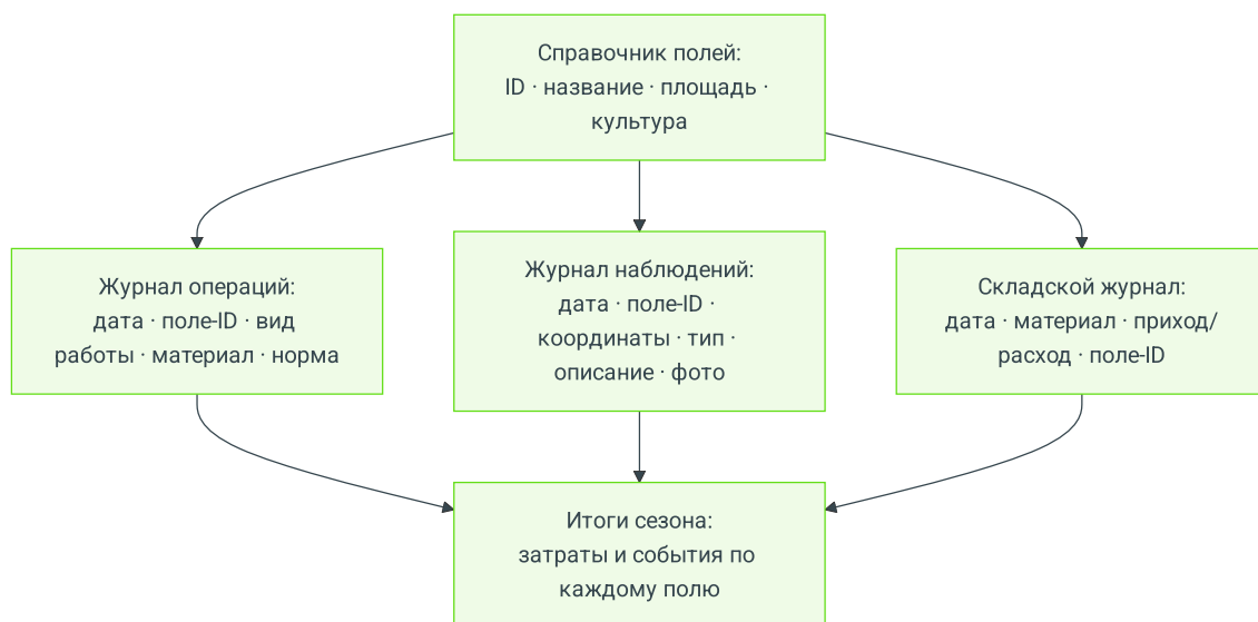
Рис. 1. Справочник полей — скелет системы учёта: все журналы ссылаются на ID поля, и только поэтому данные сезона можно свести воедино. Alt: схема — блок «Справочник полей» соединён стрелками с тремя журналами (операций, наблюдений, складским), каждый из которых содержит колонку «поле-ID»; все три журнала сходятся в блок «Итоги сезона по каждому полю».
