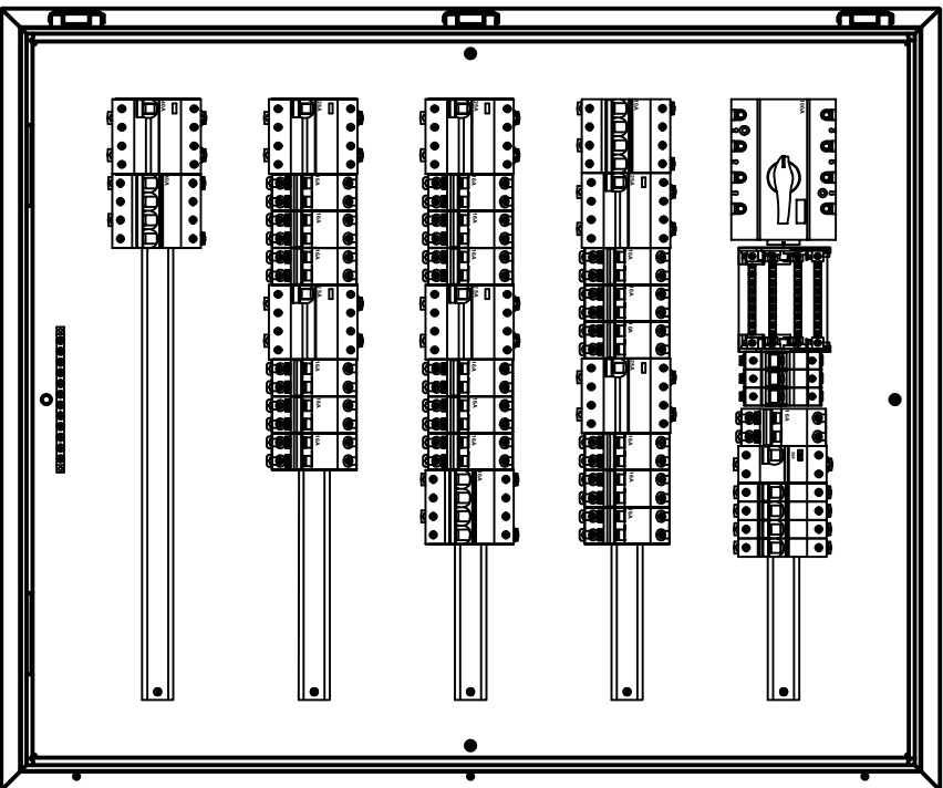
VISTA FRONTAL SIN PUERTA CON BANDEJA
