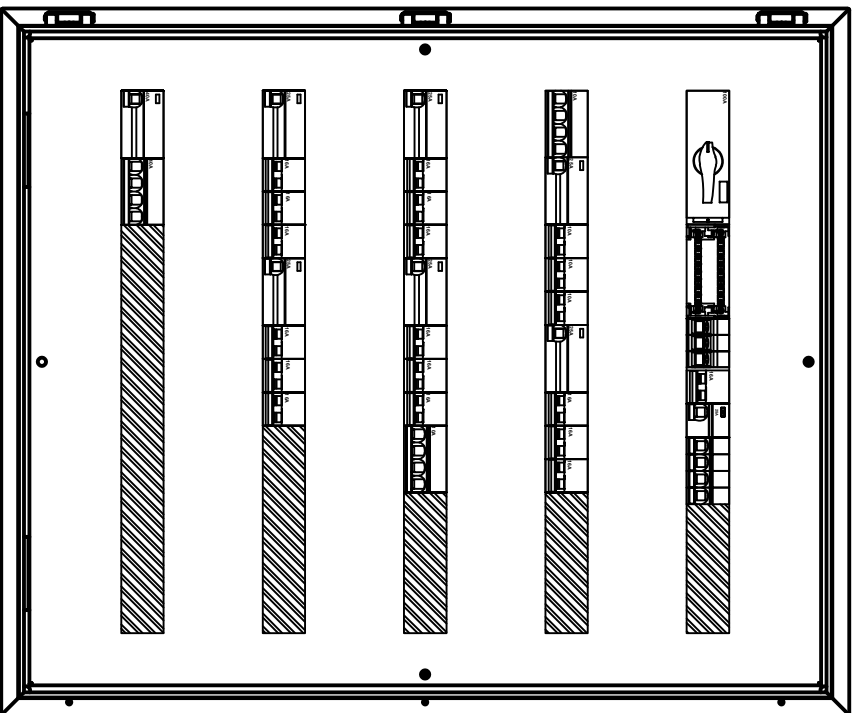
VISTA FRONTAL SIN PUERTA CON CONTRAFRENTE
