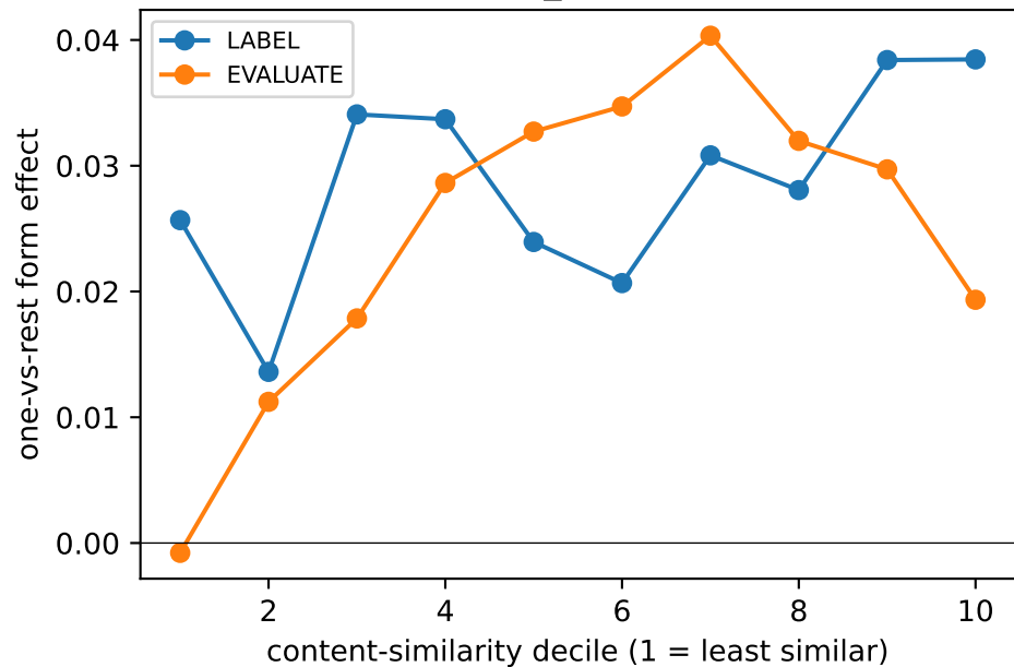
pos_cosine
