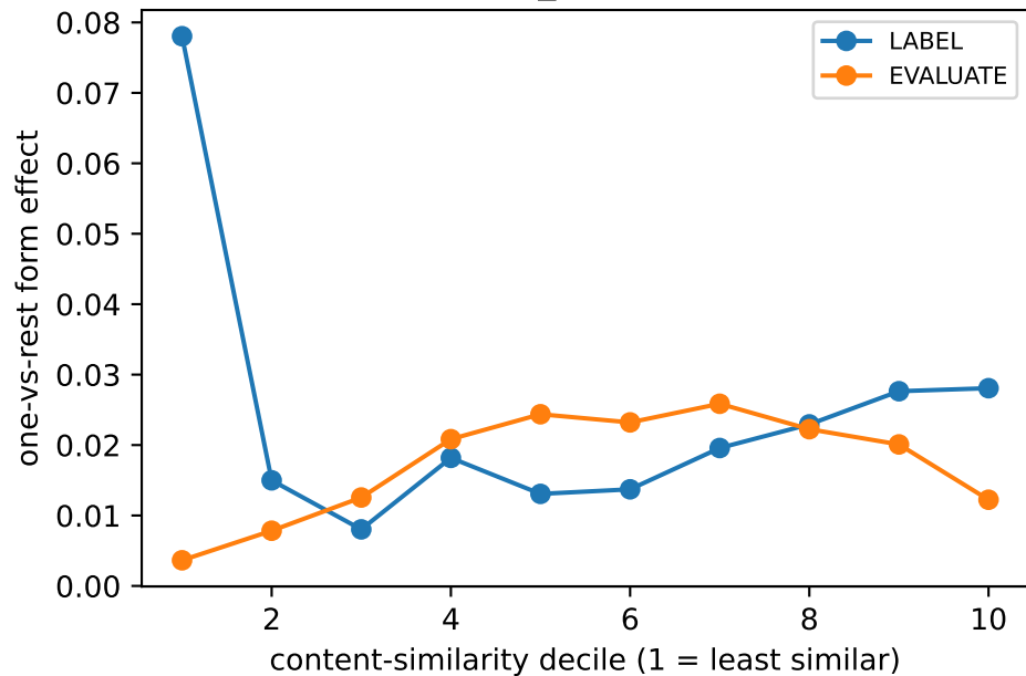
fw_negjsd
