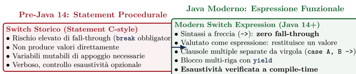
Figura 1.5: Confronto architetturale tra switch statement storico e moderna switch expression.
