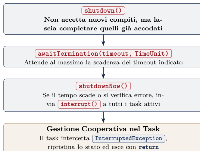
Figura 5.4: Protocollo a 4 stadi per la chiusura sicura di un ExecutorService ( ThreadApp03 ).
