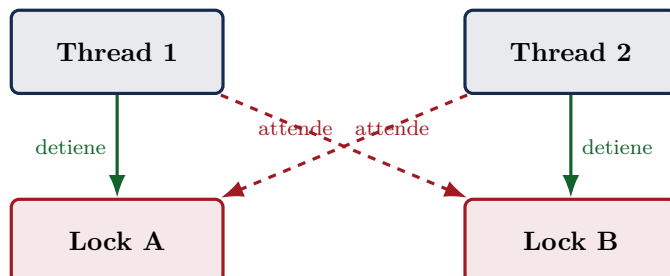
Figura 5.6: Lo stallo circolare del Deadlock: dipendenza ciclica tra lock e thread.
