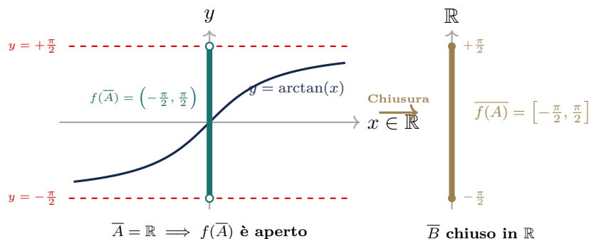
Figura 2.3: Controesempio alla commutazione tra chiusura e mappa continua: per f(x) = \arctan(x) con A = \mathbb{R} (chiuso), l'immagine è l'aperto f(\bar{A}) = (-\pi/2, \pi/2) , mentre la sua chiusura \overline{f(A)} = [-\pi/2, \pi/2] include i punti asintotici \pm\pi/2 , provando che in generale f(\bar{A}) \subsetneq \overline{f(A)} .
