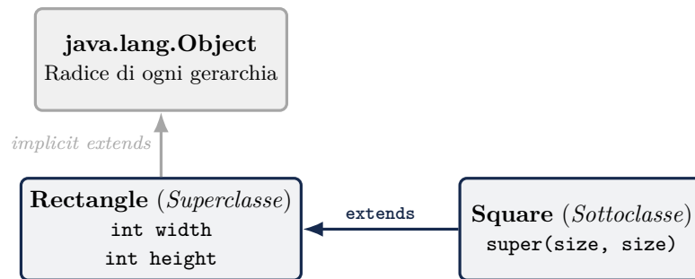
Figura 1.2: Gerarchia di ereditarietà tra Square e Rectangle , con derivazione da Object .
