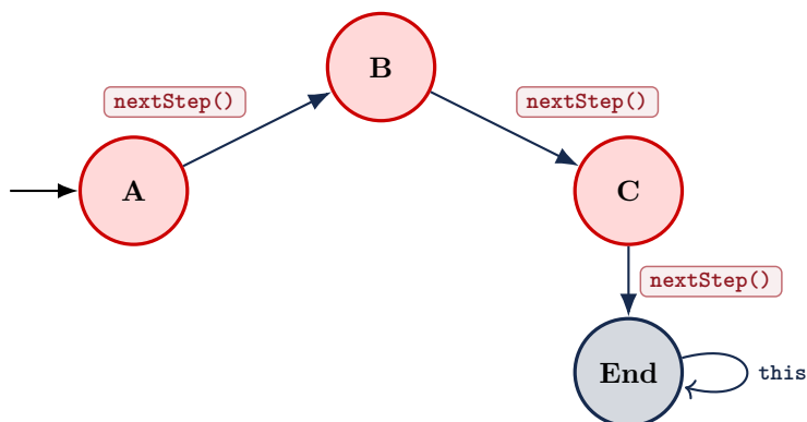
Figura 1.6: Diagramma di transizione degli stati della Macchina a Stati Finiti modellata con enum Java.
