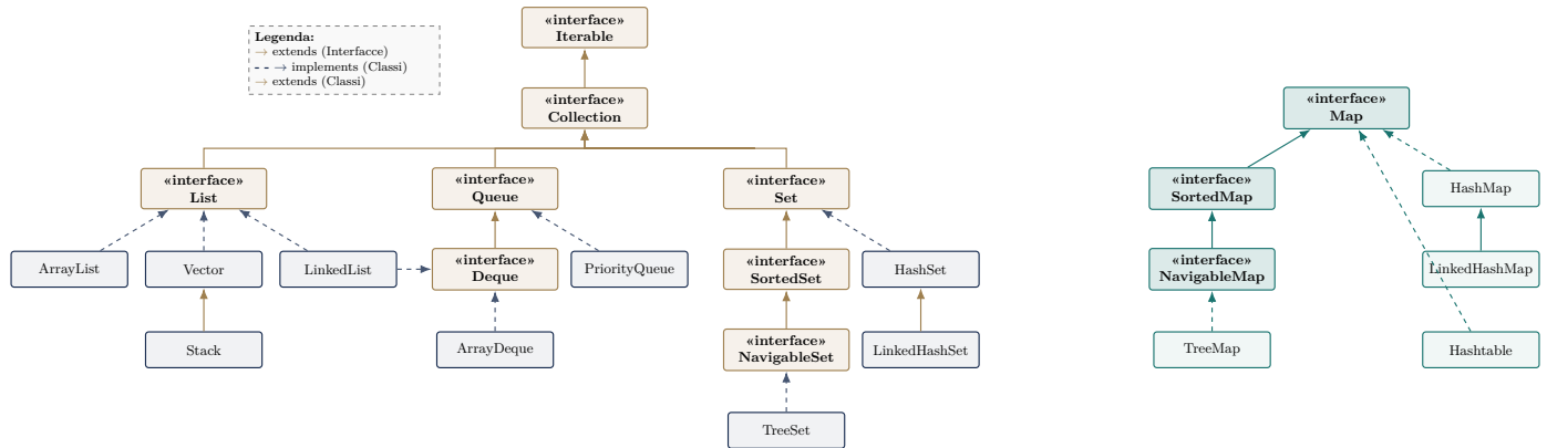
Figura 1.4: Tassonomia fondamentale del Java Collections Framework (le Mappe costituiscono una gerarchia indipendente da Collection ).
