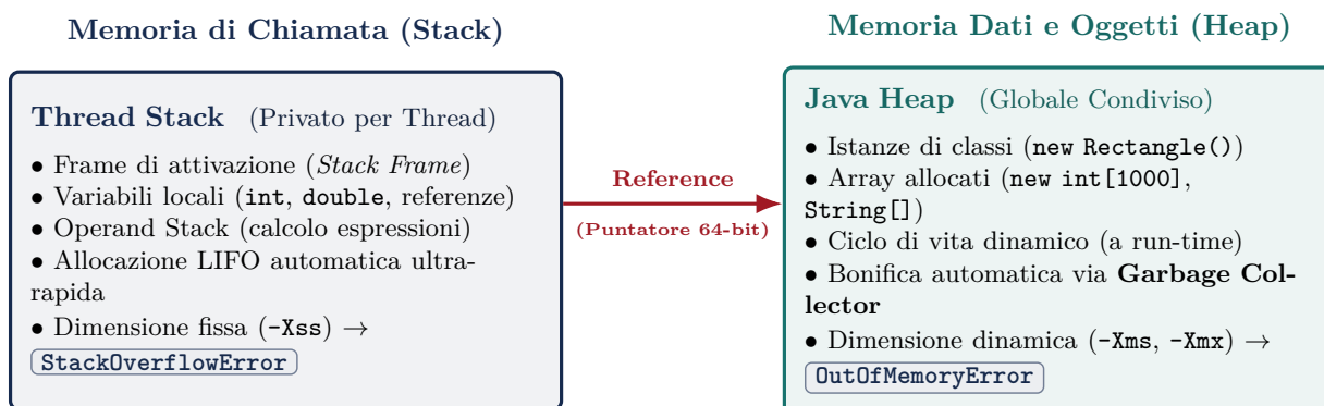
Figura 1.1: Disaccoppiamento strutturale della memoria Java: Stack privato dei thread vs Heap condiviso.
