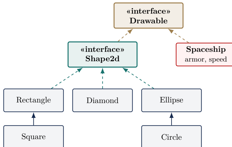
Figura 1.3: Diagramma architetturale completo: separazione semantica tra forme geometriche («Shape2d») e protocollo visivo («Drawable»).
