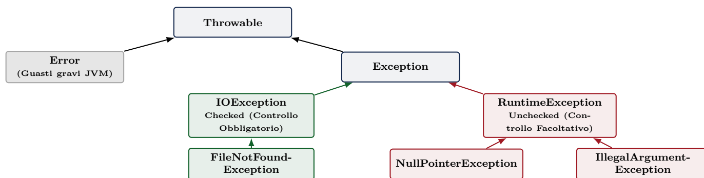
Figura B.2: Gerarchia delle eccezioni in Java: distinzione tra Checked (obbligo di gestione) e Unchecked.
