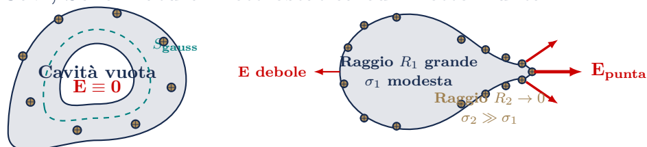
(a) Conduttore cavo (Gabbia di Faraday) (b) Effetto punta ( \sigma \propto 1/R )
