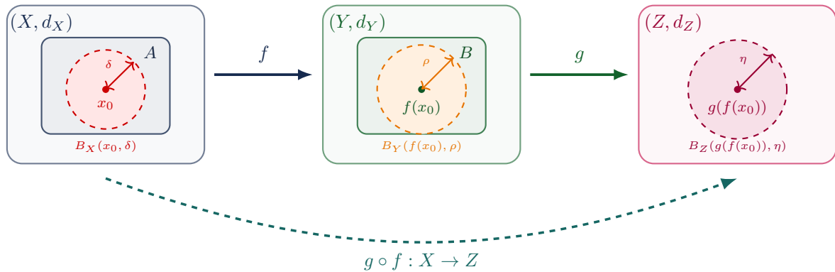
Figura 2.8: Schema della continuità della composizione: assegnato \eta > 0 in Z , la continuità di g determina \rho > 0 in Y , che a sua volta determina tramite la continuità di f il raggio \delta > 0 in X .
