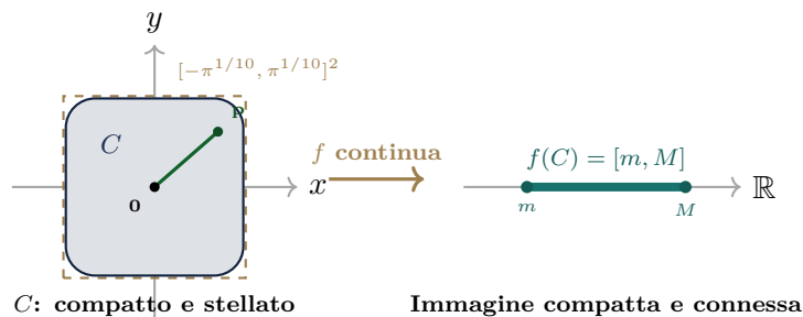
Figura 2.4: Mappatura del dominio decico C = \{x^{10} + y^{10} \leq \pi\} : compatto (chiuso e limitato da [-\pi^{1/10}, \pi^{1/10}]^2 ) e connesso per archi (stellato rispetto all'origine). Per i teoremi di Weierstrass e dei valori intermedi, f(C) è compatto e connesso in \mathbb{R} , ossia un intervallo chiuso e limitato [m, M] .
