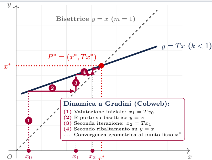
Figura 2.11: Significato geometrico della contrazione: la curva y = Tx , avente pendenza uniformemente minore di 1 ( k < 1 ), incontra la bisettrice y = x in un unico punto fisso x^* . L'iterazione x_{n+1} = Tx_n produce quindi una successione che converge a x^* con velocità geometrica di ragione k .
