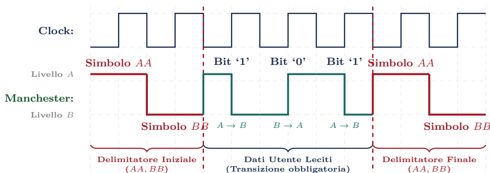
Figura 3.6: Cronogramma delle violazioni di codifica fisica su codifica Manchester: i bit leciti ('0' e '1') presentano sempre una transizione di livello a centro periodo, mentre i simboli costanti senza transizione (AA e BB) sono violazioni intenzionali impiegate per delimitare la trama.
