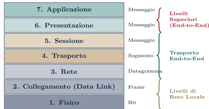
Figura 2.9: I sette livelli del modello ISO/OSI con le relative PDU. I livelli 5-7 risiedono esclusivamente sugli host end-to-end; il livello 3 governa l'instradamento nella rete; i livelli 1-2 operano tra nodi direttamente adiacenti.
