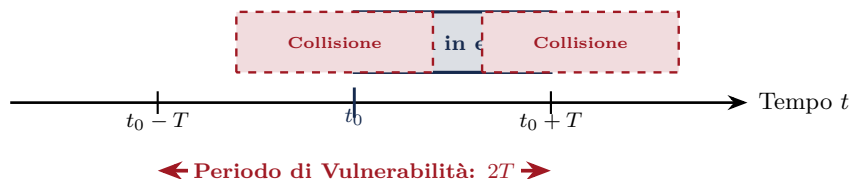
Figura 3.12: Periodo di vulnerabilità del protocollo ALOHA puro: affinché la trama trasmessa nell'intervallo [t_0, t_0 + T] abbia successo, nessun'altra trama deve essere emessa nell'intervallo [t_0 - T, t_0 + T] , di estensione complessiva pari a 2T .
