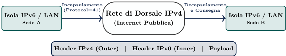
Figura 2.12: Architettura di tunneling IPv6-in-IPv4 (Protocollo 41): le sedi remote comunicano in modo trasparente attraverso la rete IPv4.
