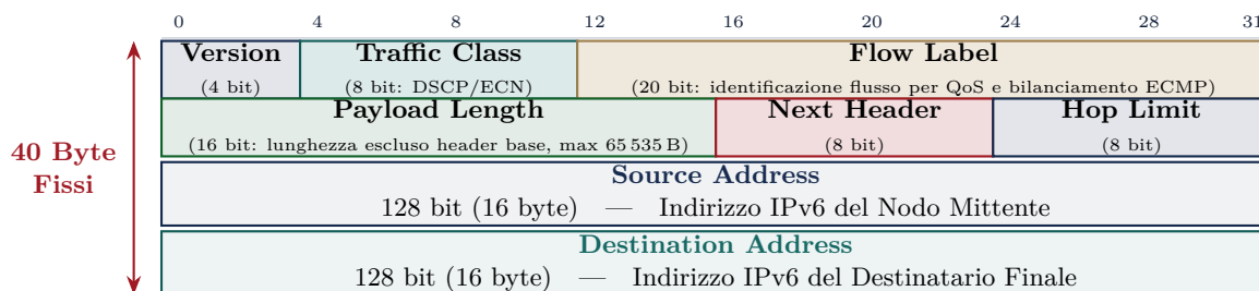
Figura 2.22: Struttura e campi dell'Header Base IPv6 a 40 byte fissi (RFC 8200).
