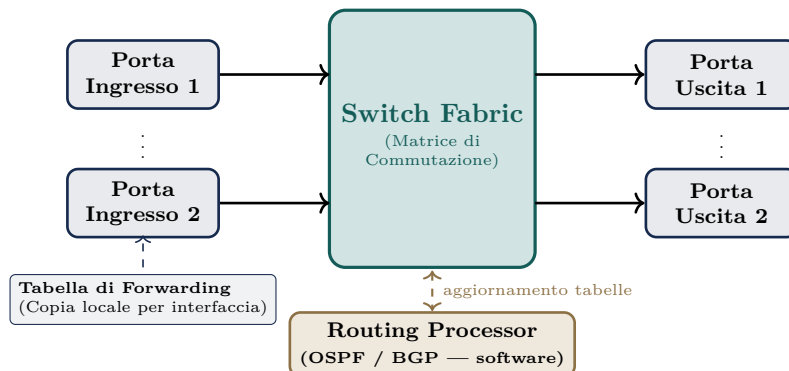
Figura 2.20: Architettura interna di un router: separazione tra il piano dati ad alta velocità (line card di ingresso/uscita e matrice di commutazione) e il piano di controllo software (Routing Processor).
