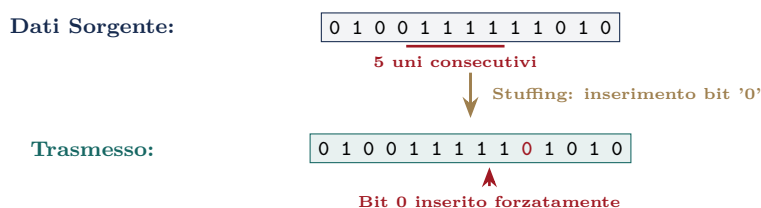
Figura 3.5: Meccanismo del Bit Stuffing: inserimento forzato di uno '0' dopo cinque '1' consecutivi per preservare l'univocità del flag.
