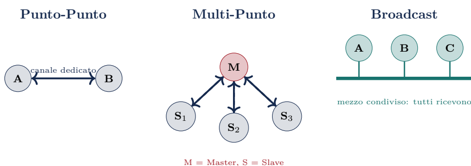
Figura 2.3: Tipologie di canale: punto-punto (risorse dedicate), multi-punto (master/slave con arbitraggio), broadcast (mezzo condiviso).
