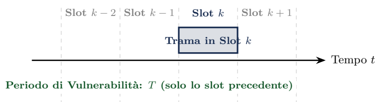
Figura 3.13: Periodo di vulnerabilità di Slotted ALOHA: la discretizzazione temporale vincola le trasmissioni all'inizio degli slot, dimezzando la vulnerabilità a un singolo tempo di trama T .
