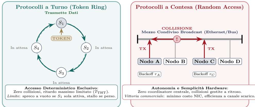
Figura 3.11: Confronto concettuale tra le due filosofie di allocazione dinamica del canale (§3.9.1 vs §3.9.2): a sinistra, i Protocolli a Turno (Token Ring) , in cui l'accesso è rigidamente coordinato dalla circolazione deterministica di un gettone logico che previene alla radice le collisioni al prezzo di complessità e latenza; a destra, i Protocolli a Contesa (Random Access) , fondati su stazioni autonome che accedono spontaneamente al mezzo condiviso e risolvono le inevitabili collisioni tramite algoritmi probabilistici di backoff.
