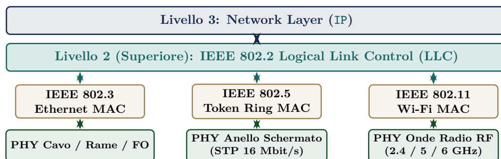
Figura 3.10: Architettura standard IEEE 802: disaccoppiamento tra il sottolivello superiore LLC (comune e indipendente dal mezzo) e il sottolivello inferiore MAC (specifico per ciascuna tecnologia di canale condiviso).
