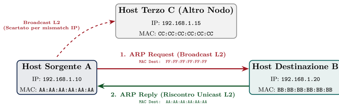
Figura 3.21: Flusso operativo del protocollo ARP: interrogazione broadcast di Livello 2 e riscontro unicast diretto dal nodo destinatario.
