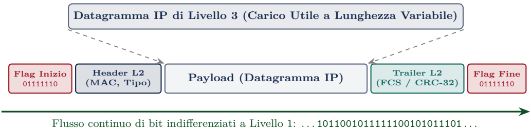
Figura 3.4: Incapsulamento del datagramma IP nella trama di Livello 2 e sua proiezione sul flusso continuo di bit di Livello 1.
