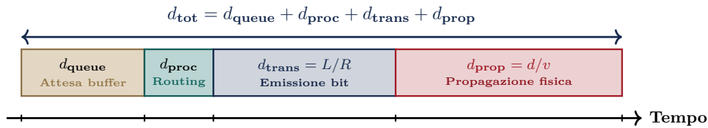
Figura 2.2: Scomposizione del ritardo nodale in un router: le quattro componenti additive. Il ritardo di accodamento è variabile e dipende dal carico istantaneo; il ritardo di propagazione è deterministico e dipende dalla distanza fisica.
