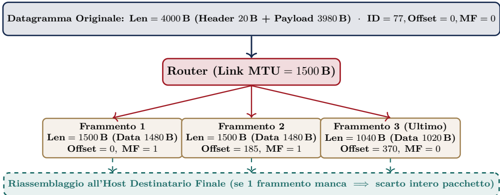
Figura 2.13: Processo di frammentazione IP: calcolo degli offset multipli di 8 byte e gestione dei flag MF.
