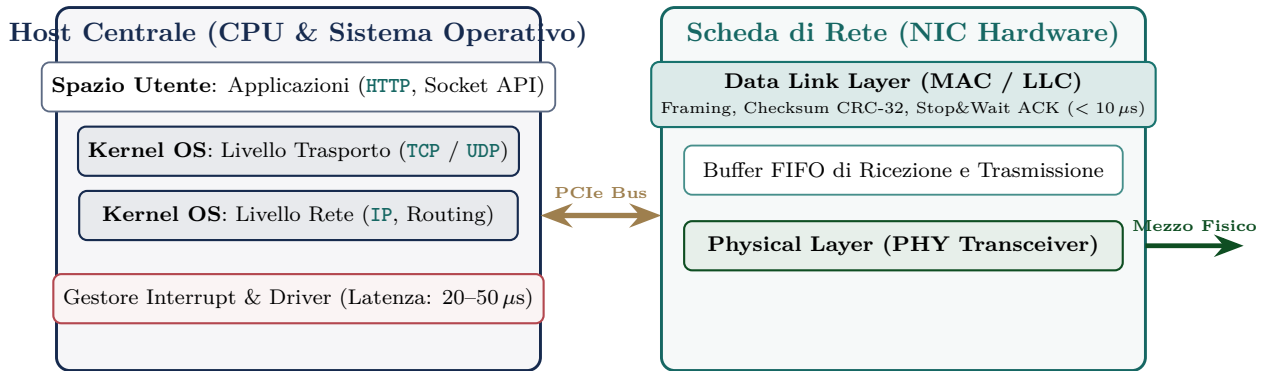
Figura 3.2: Ripartizione architetturale tra le funzioni software gestite dalla CPU nel kernel del sistema operativo (Livelli 3 e 4) e le funzioni in tempo reale eseguite in hardware a bordo della scheda di rete (NIC, Livelli 1 e 2).
