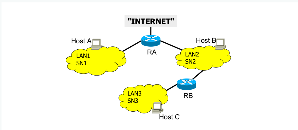
Figura 2.21: Topologia ufficiale della rete di campus con tre zone (LAN1, LAN2, LAN3), router R_A ed R_B , collegamento ISP /30 e host A, B, C (Esercizio 5).
