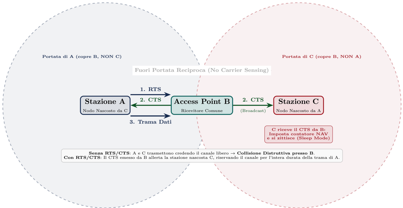
Figura 3.19: Il Problema del Terminale Nascosto ( Hidden Node ) nelle reti Wi-Fi e sua risoluzione tramite handshake a quattro vie (RTS/CTS). Le stazioni A e C non possono avvertirsi reciprocamente; l'Access Point intermedio B trasmette il Clear to Send (CTS) in broadcast, consentendo a C di acquisire la durata dell'occupazione e impostare il proprio Network Allocation Vector (NAV) per congelarsi durante la trasmissione di A.
