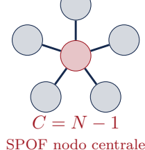
Figura 2.4: Topologie di rete fondamentali a confronto: formule di connettività C e caratteristiche di affidabilità.
