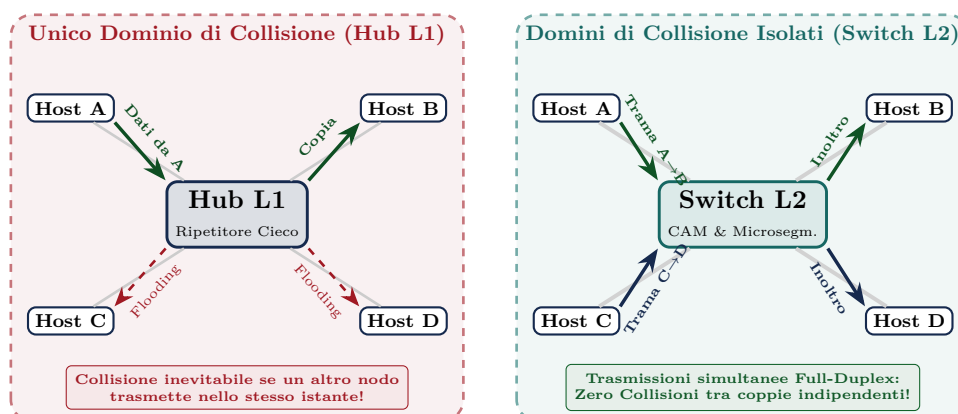
Figura 3.16: Confronto architetturale tra Hub (Livello 1) e Switch (Livello 2): l'Hub replica ciecamente i segnali generando un unico dominio di collisione condiviso; lo switch isola ciascuna porta in un dominio di collisione indipendente permettendo trasmissioni parallele e full-duplex privo di contesa.
