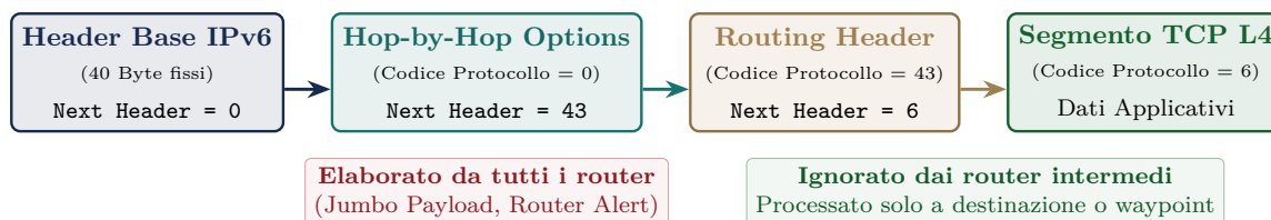
Figura 2.23: Principio del Daisy-Chaining degli Extension Headers con puntatori Next Header.
