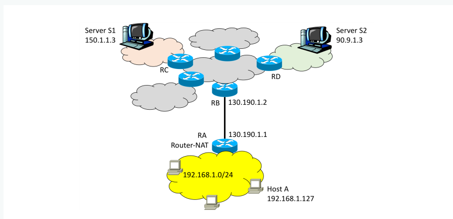
Figura 2.19: Topologia ufficiale della subnet privata attestata a Internet con Router-NAT R_A , router di transito R_B , R_C , R_D e server remoti S_1 , S_2 (Esercizio 4).
