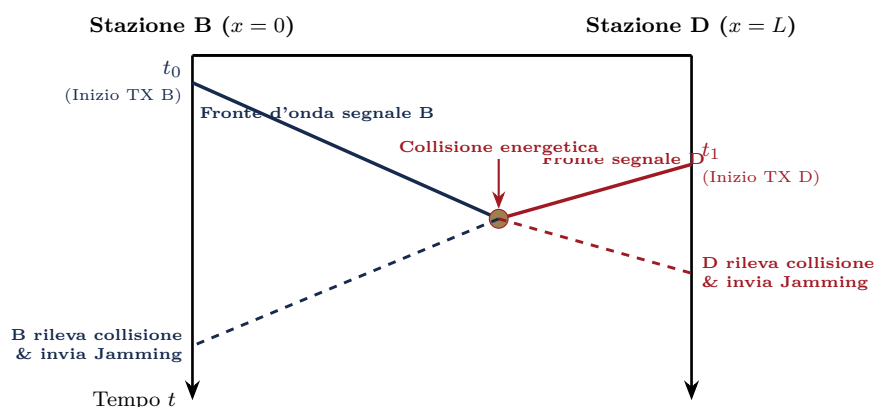
Figura 3.15: Diagramma spazio-temporale della collisione tra due stazioni Ethernet ( B e D ) su bus condiviso: D inizia a trasmettere a t_1 prima che il segnale di B la raggiunga. La collisione viene rilevata in istanti differenti; l'emissione della Jamming Sequence garantisce che la sovrapposizione energetica raggiunga entrambe le stazioni.
