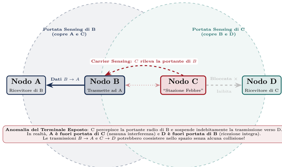
Figura 3.20: Il Problema del Terminale Esposto ( Exposed Node ) nelle reti radio locali. Il nodo C (la “stazione con la febbre”) avverte l’energia elettromagnetica della trasmissione B \rightarrow A e sospende indebitamente l’invio verso D, sebbene il ricevitore D sia immune all’interferenza di B e il ricevitore A sia oltre la portata di C, causando uno spreco di capacità spaziale del canale.
