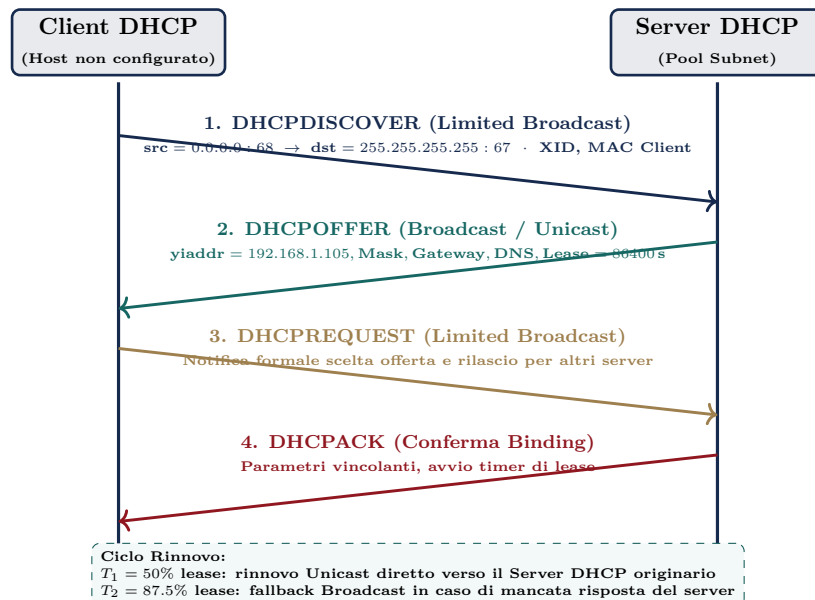
Figura 2.16: Ladder diagram del processo di configurazione a quattro vie ( 4-Way Handshake DORA ) in DHCP.
