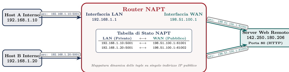
Figura 2.17: Architettura NAPT: due host con medesima porta sorgente interna (5001) vengono multiplexati su porte pubbliche distinte (61001 e 61002) verso il medesimo server HTTP.
