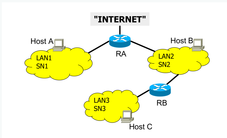
Figura 2.14: Topologia ufficiale della rete di campus: LAN1, LAN2 e LAN3 separate dai router R_A ed R_B , con accesso Internet da R_A e posizionamento degli Host A, B e C.
