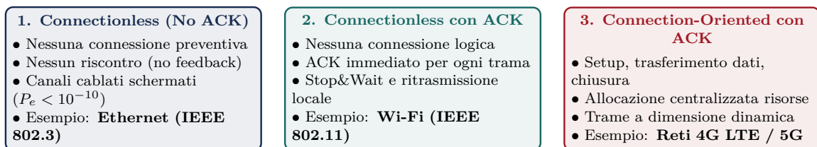
Figura 3.3: Tassonomia delle tre classi di servizio offerte dal Livello 2 al protocollo di rete IP.
