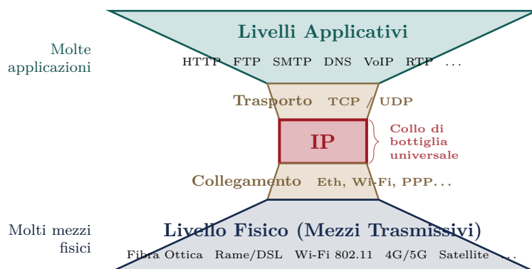
Figura 1.1: L'architettura a clessidra di Internet: la varietà dei mezzi fisici (basso) e dei protocolli applicativi (alto) converge sull'unico denominatore comune IP, che rimane invariato.
