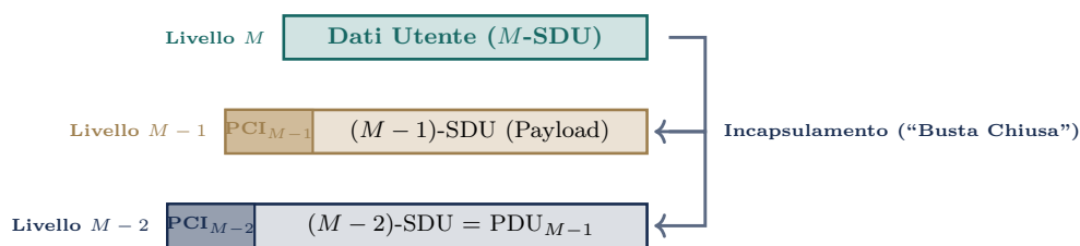
Figura 2.8: Il meccanismo dell'incapsulamento: ogni livello tratta la PDU ricevuta dallo strato superiore come una SDU (busta chiusa opaca), prefiggendovi la propria intestazione di controllo (PCI).
