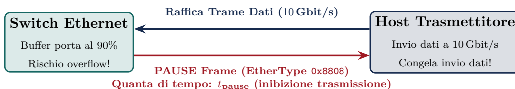
Figura 3.9: Controllo di flusso Ethernet Full-Duplex (IEEE 802.3x): lo switch invia un PAUSE Frame per arrestare temporaneamente il trasmettitore ed evitare l'overflow dei buffer interni.
