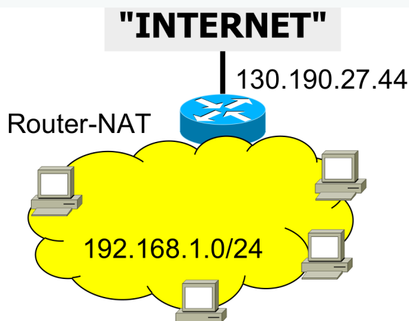
Figura 2.18: Topologia ufficiale della subnet privata attestata a Internet tramite il Router-NAT con interfaccia esterna 130.190.27.44/28.
