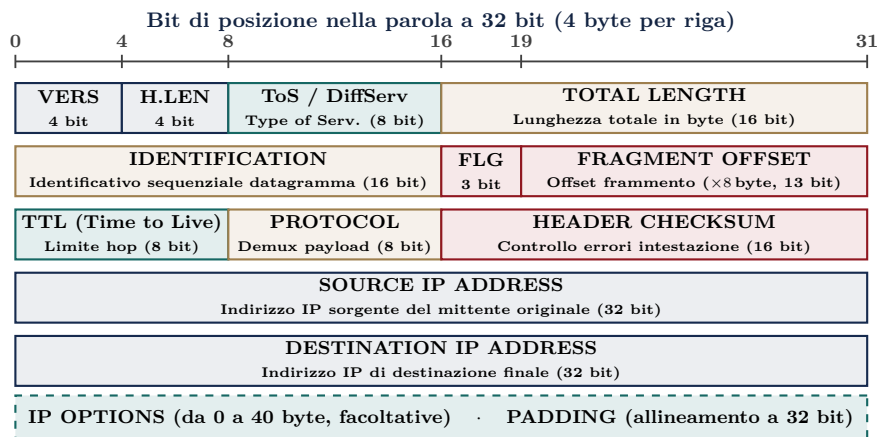
Figura 2.11: Struttura dell'intestazione IPv4 (RFC 791). La testata minima priva di opzioni misura esattamente 20 byte (5 parole da 32 bit).
