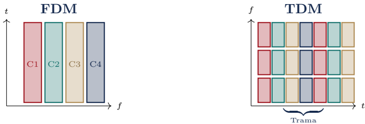
Figura 2.5: Commutazione di circuito: allocazione FDM (banda di frequenza fissa) e TDM (slot temporale fisso). In entrambi i casi le risorse sono riservate per l’intera durata della comunicazione.
