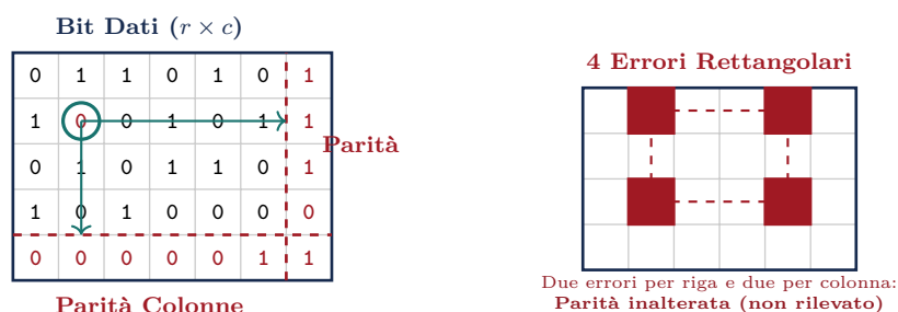
Figura 3.7: A sinistra: correzione hardware dell'errore singolo all'intersezione riga-colonna. A destra: il pattern di 4 errori ai vertici di un rettangolo che elude completamente il controllo.
