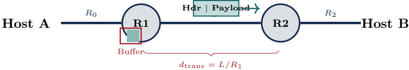
Figura 2.6: Store-and-Forward: il router R1 riceve l’intero pacchetto prima di iniziare a trasmetterlo sul link successivo. Il ritardo totale su k hop è k \cdot L/R (trascurando propagazione e accodamento).
