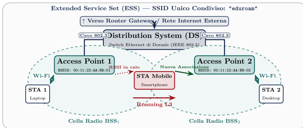
Figura 3.17: Architettura di una rete WLAN IEEE 802.11 in modalità infrastruttura: l'Extended Service Set (ESS) raggruppa celle elementari (BSS 1 e BSS 2 ) identificate dallo stesso SSID logico. Gli Access Point commutano il traffico verso la dorsale cablata (Distribution System), garantendo il roaming continuo dei terminali senza interruzione della sessione IP.
