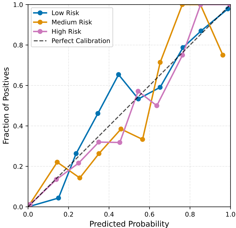
Calibration Plot: Model Confidence vs. Actual Outcomes
